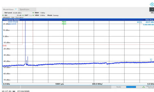
NTV-n77(3450-3550)-PC1.5-30-50-L-DFT-BPSK-Inner_1RB_Left-3000-6000-PASS
