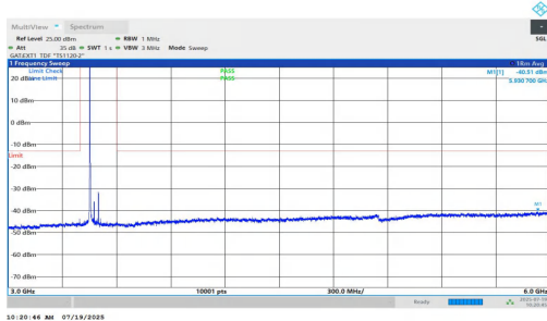
NTNV-n77(3450-3550)-PC1.5-30-50-L-DFT-QPSK-Inner_1RB_Left-3 000-6000-PASS
