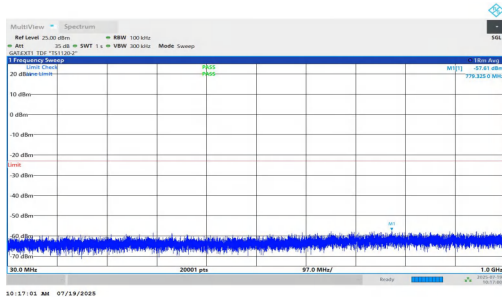
NTV-n77(3450-3550)-PC1.5-30-50-L-DFT-BPSK-Inner_1RB_Left-30-1000-PASS
