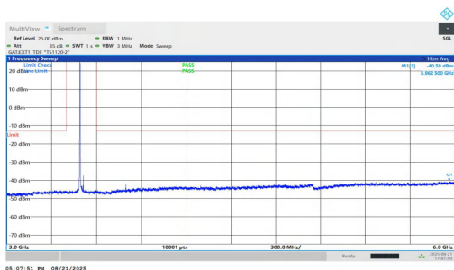
NTNV-n77(3450-3550)-PC1.5-30-25-M-DFT-QPSK-Inner_1RB_Left-3 000-6000-PASS
