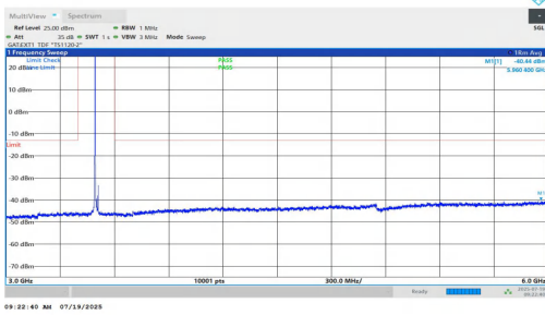
NTVN-n77(3450-3550)-PC1.5-30-20-M-DFT-BPSK-Inner_1RB_Left-3 000-6000-PASS
