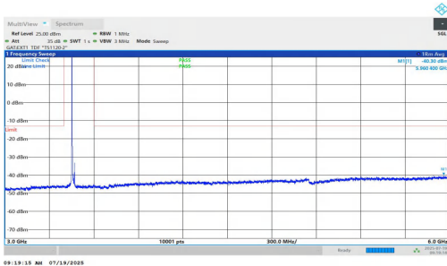
NTNV-n77(3450-3550)-PC1.5-30-20-L-DFT-QPSK-Inner_1RB_Left-3 000-6000-PASS
