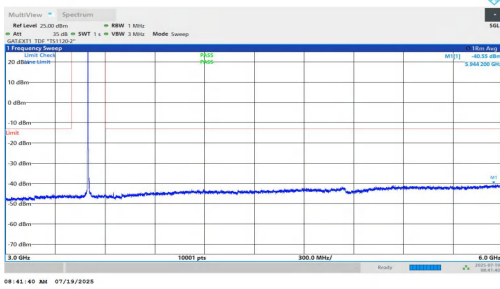
NTV-n77(3450-3550)-PC1.5-30-10-M-DFT-BPSK-Inner_1RB_Left-3 000-6000-PASS
