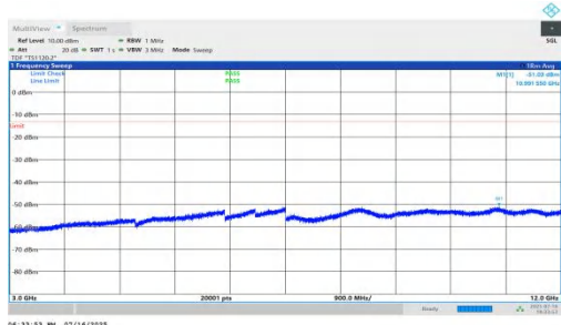
NTNV-n71-PC2-15-20-L-DFT-QPSK-Inner_1RB_Left-3000-12000-PA SS
