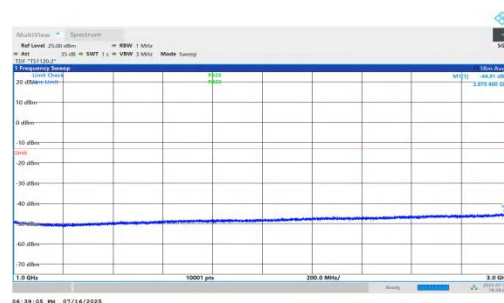
NTNV-n71-PC2-15-20-H-DFT-QPSK-Inner_1RB_Left-1000-3000-PAS
