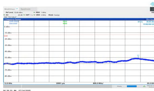
NTNV-n71-PC2-15-20-M-DFT-BPSK-Inner_1RB_Right-12000-20000-P ASS
