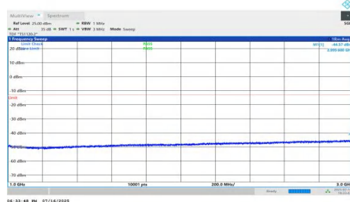
NTNV-n71-PC2-15-20-L-DFT-QPSK-Inner_1RB_Left-1000-3000-PASS
