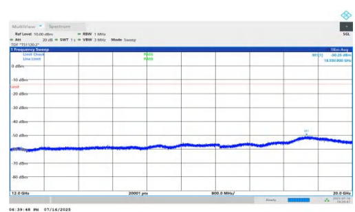
NTNV-n71-PC2-15-20-H-DFT-QPSK-Inner_1RB_Right-12000-20000-P ASS
