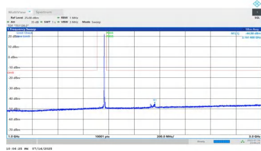
NTNV-n66-PC2-15-40-M-DFT-QPSK-Inner_1RB_Right-1000-3000- -PASS
