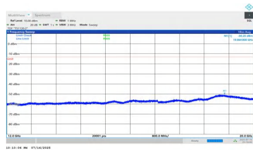
NTNV-n66-PC2-15-45-L-DFT-BPSK-Inner_1RB_Left-12000-20000 -PASS
