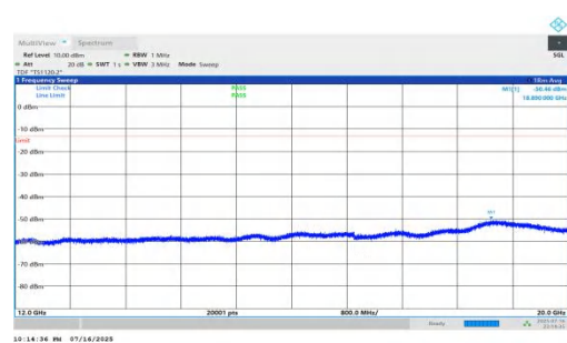
NTNV-n66-PC2-15-45-M-DFT-QPSK-Inner_1RB_Right-12000-200 00-PASS
