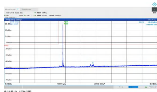
NTNV-n66-PC2-15-45-M-DFT-QPSK-Inner_1RB_Right-1000-3000 -PASS
