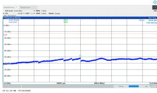
NTVN-n66-PC2-15-45-L-DFT-QPSK-Inner_1RB_Left-3000-12000 -PASS
