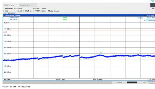
NTVN-n66-PC2-15-25-L-DFT-QPSK-Inner_1RB_Left-3000-12000 -PASS
