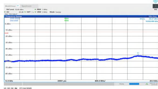
NTNV-n66-PC2-15-40-L-DFT-BPSK-Inner_1RB_Left-12000-20000 -PASS
