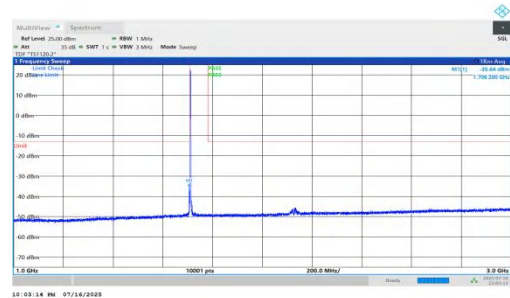
NTNV-n66-PC2-15-40-L-DFT-QPSK-Inner_1RB_Left-1000-3000-P ASS
