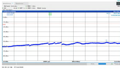
NTV-n66-PC2-15-35-L-DFT-QPSK-Inner_1RB_Left-3000-12000 -PASS
