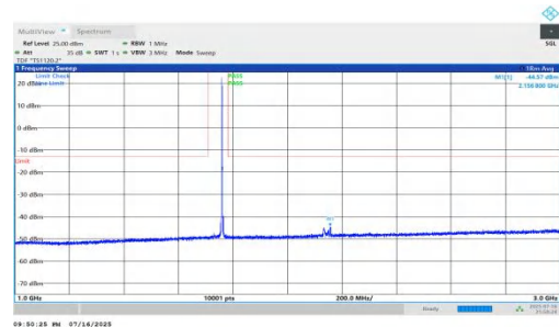
NTNV-n66-PC2-15-30-M-DFT-QPSK-Inner_1RB_Right-1000-3000- -PASS
