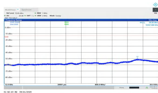
NTNV-n66-PC2-15-25-M-DFT-QPSK-Inner_1RB_Right-12000-200 00-PASS
