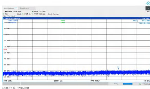
NTNV-n66-PC2-15-40-L-DFT-QPSK-Inner_1RB_Left-30-1000-PA SS
