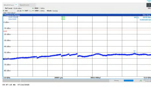
NTV-n66-PC2-15-30-L-DFT-QPSK-Inner_1RB_Left-3000-12000 -PASS
