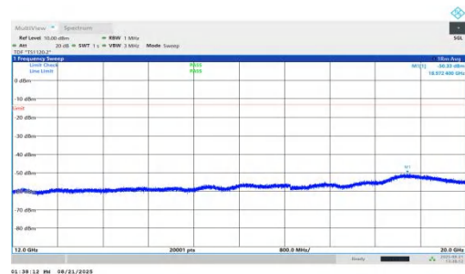
NTNV-n66-PC2-15-25-L-DFT-BPSK-Inner_1RB_Left-12000-20000 -PASS
