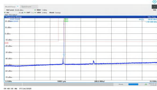
NTNV-n66-PC2-15-20-H-DFT-QPSK-Inner_1RB_Right-1000-3000 -PASS
