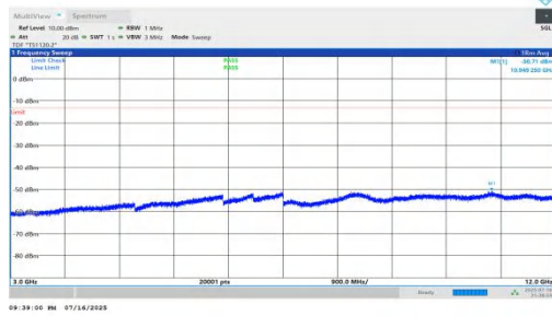
NTVN-n66-PC2-15-20-L-DFT-QPSK-Inner_1RB_Left-3000-12000 -PASS
