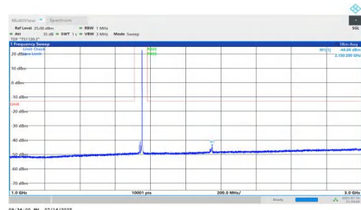
NTNV-n66-PC2-15-15-M-DFT-QPSK-Inner_1RB_Right-1000-3000 -PASS
