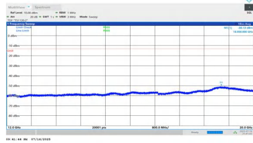
NTNV-n66-PC2-15-20-M-DFT-QPSK-Inner_1RB_Left-12000-2000 0-PASS
