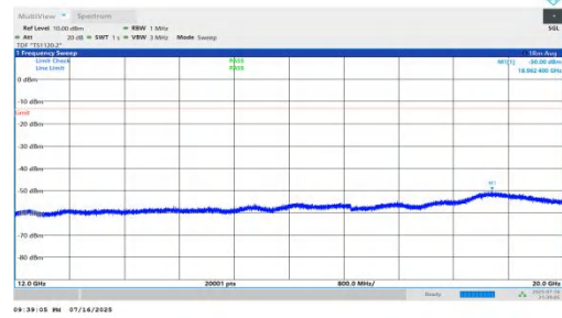
NTVN-n66-PC2-15-20-L-DFT-QPSK-Inner_1RB_Left-12000-2000 0-PASS
