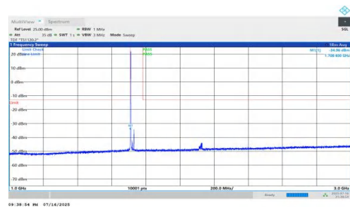
NTNV-n66-PC2-15-20-L-DFT-QPSK-Inner_1RB_Left-1000-3000-P ASS
