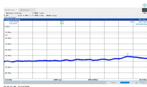
NTVN-n66-PC2-15-20-L-DFT-QPSK-Inner_1RB_Right-12000-20000- 00-PASS
