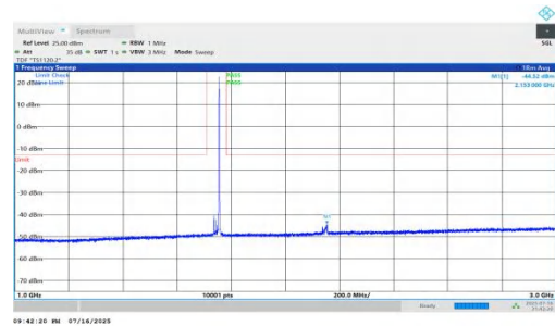
NTNV-n66-PC2-15-20-M-DFT-QPSK-Inner_1RB_Right-1000-3000 -PASS
