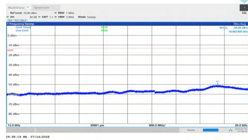
NTNV-n66-PC2-15-20-L-DFT-BPSK-Inner_1RB_Right-12000-200 00-PASS
