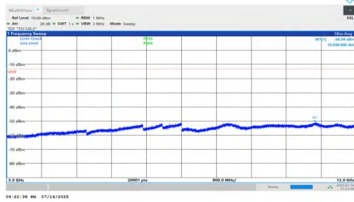
NTNV-n66-PC2-15-10-L-DFT-QPSK-Inner_1RB_Left-3000-12000 -PASS
