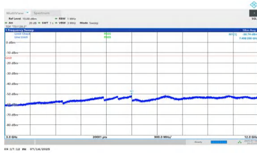
NTNV-n66-PC2-15-5-M-DFT-QPSK-Inner_1RB_Left-3000-12000 -PASS
