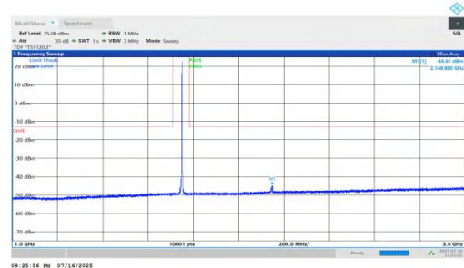
NTNV-n66-PC2-15-10-M-DFT-QPSK-Inner_1RB_Right-1000-3000- -PASS
