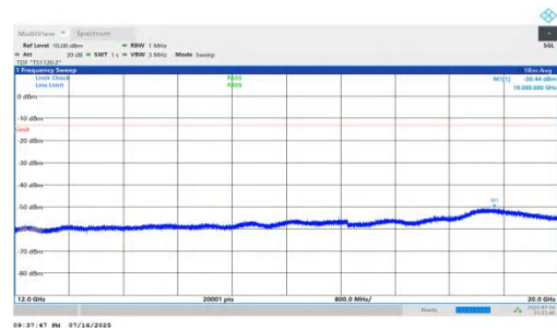
NTNV-n66-PC2-15-20-L-DFT-BPSK-Inner_1RB_Left-12000-20000-PASS
