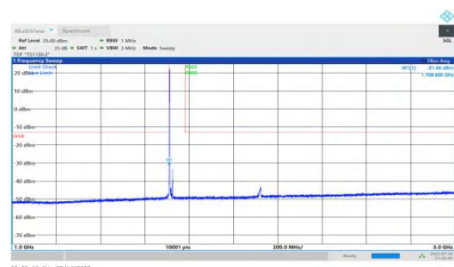
NTNV-n66-PC2-15-15-L-DFT-QPSK-Inner_1RB_Left-1000-3000-P ASS
