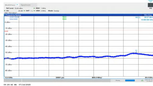
NTNV-n66-PC2-15-15-L-DFT-BPSK-Inner_1RB_Left-12000-20000 -PASS
