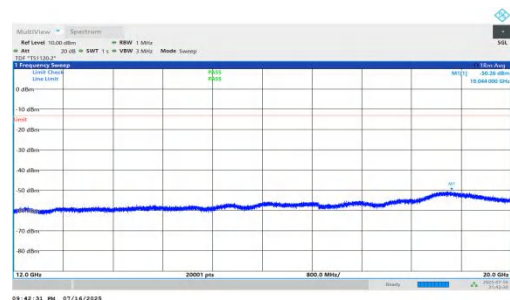
NTNV-n66-PC2-15-20-M-DFT-QPSK-Inner_1RB_Right-12000-200 00-PASS
