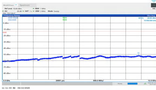
NTNV-n66-PC3-15-45-L-DFT-QPSK-Inner_1RB_Left-3000-12000 -PASS
