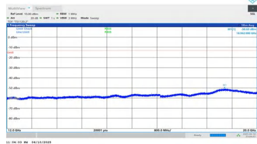
NTNV-n66-PC3-15-40-L-DFT-QPSK-Inner_1RB_Right-12000-200 00-PASS
