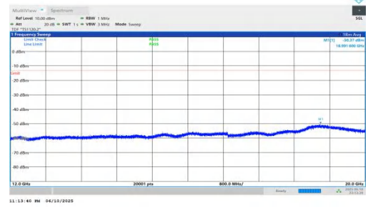
NTNV-n66-PC3-15-45-M-DFT-QPSK-Inner_1RB_Left-12000-2000 0-PASS
