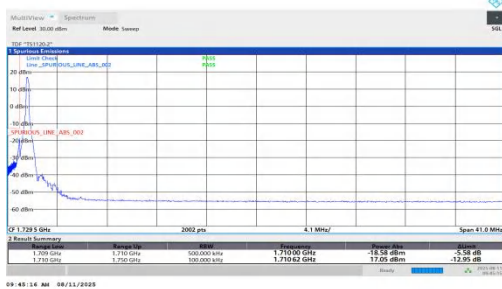
NTNV-n66-PC2-15-40-L-DFT-QPSK-Edge_1RB_Left-PASS
