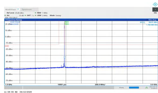
NTNV-n66-PC3-15-40-H-DFT-QPSK-Inner_1RB_Right-1000-3000 -PASS
