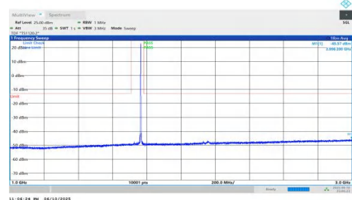
NTNV-n66-PC3-15-40-M-DFT-QPSK-Inner_1RB_Right-1000-3000- -PASS
