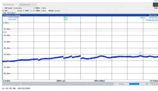
NTNV-n66-PC3-15-45-M-DFT-QPSK-Inner_1RB_Left-3000-1200 0-PASS
