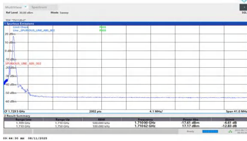
NTNV-n66-PC2-15-40-L-DFT-BPSK-Edge_1RB_Left-PASS
