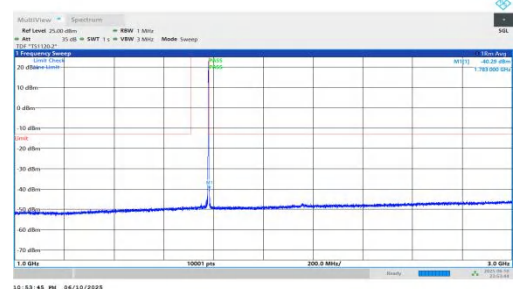
NTNV-n66-PC3-15-30-H-DFT-QPSK-Inner_1RB_Right-1000-3000- -PASS
