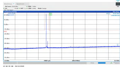
NTNV-n66-PC3-15-25-M-DFT-QPSK-Inner_1RB_Left-1000-3000-PASS
