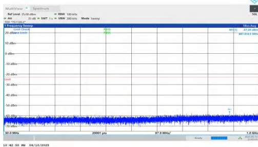
NTNV-n66-PC3-15-25-M-DFT-QPSK-Inner_1RB_Left-30-1000-PASS
