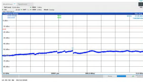
NTNV-n66-PC3-15-35-L-DFT-QPSK-Inner_1RB_Left-3000-12000 -PASS
