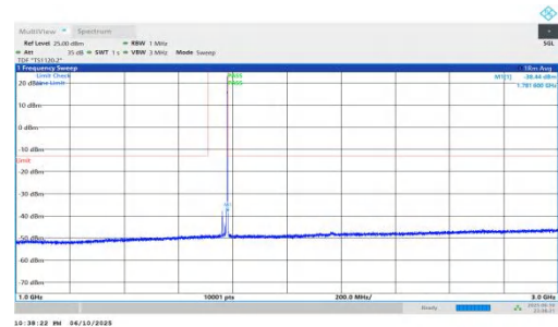
NTNV-n66-PC3-15-20-H-DFT-QPSK-Inner_1RB_Right-1000-3000 -PASS
