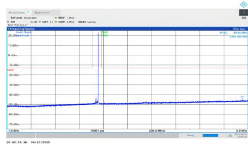
NTNV-n66-PC3-15-25-M-DFT-QPSK-Inner_1RB_Right-1000-3000- -PASS
