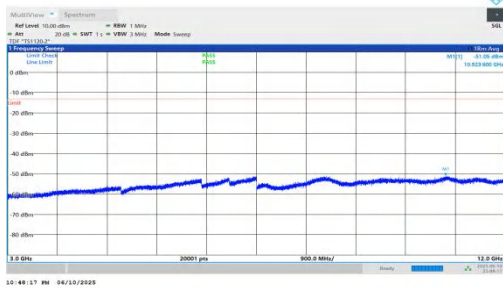
NTNV-n66-PC3-15-30-L-DFT-QPSK-Inner_1RB_Left-3000-12000 -PASS
