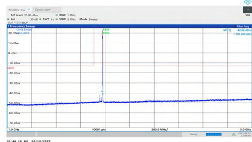
NTNV-n66-PC3-15-25-H-DFT-QPSK-Inner_1RB_Right-1000-3000 -PASS
