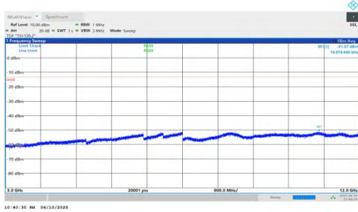
NTNV-n66-PC3-15-25-L-DFT-QPSK-Inner_1RB_Left-3000-12000 -PASS
