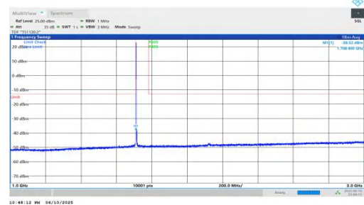
NTNV-n66-PC3-15-30-L-DFT-QPSK-Inner_1RB_Left-1000-3000-P ASS
