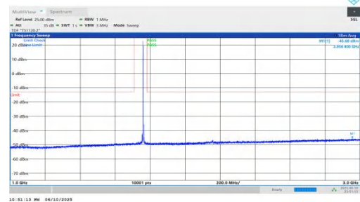
NTNV-n66-PC3-15-30-M-DFT-QPSK-Inner_1RB_Right-1000-3000- -PASS
