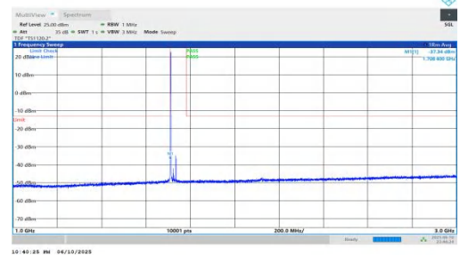
NTNV-n66-PC3-15-25-L-DFT-QPSK-Inner_1RB_Left-1000-3000-P ASS
