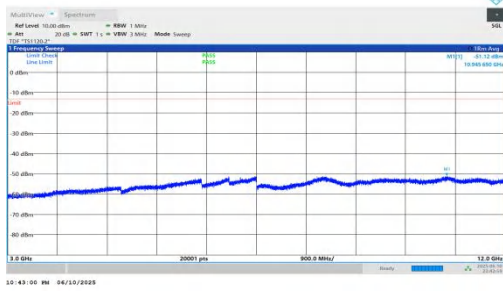
NTNV-n66-PC3-15-25-M-DFT-QPSK-Inner_1RB_Left-3000-1200 0-PASS
