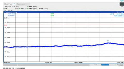
NTNV-n66-PC3-15-20-H-DFT-QPSK-Inner_1RB_Right-12000-200 00-PASS
