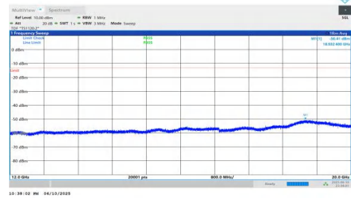
NTNV-n66-PC3-15-20-H-DFT-QPSK-Inner_1RB_Left-12000-2000 0-PASS
