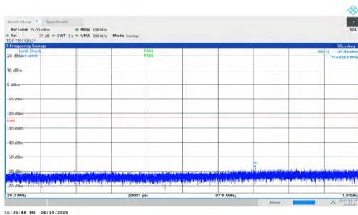
NTNV-n66-PC3-15-20-M-DFT-QPSK-Inner_1RB_Right-30-1000-PASS
