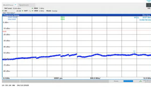
NTNV-n66-PC3-15-20-L-DFT-QPSK-Inner_1RB_Right-3000-1200 00-PASS
