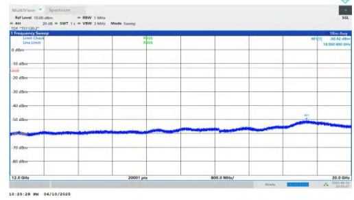
NTNV-n66-PC3-15-15-L-DFT-QPSK-Inner_1RB_Left-12000-2000 0-PASS
