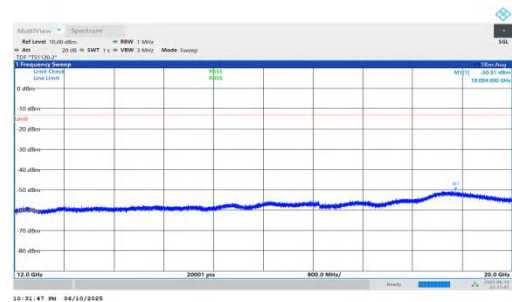
NTNV-n66-PC3-15-20-L-DFT-BPSK-Inner_1RB_Left-12000-20000-PASS
