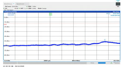
NTNV-n66-PC3-15-15-L-DFT-QPSK-Inner_1RB_Right-12000-200 00-PASS
