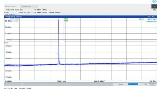
NTNV-n66-PC3-15-20-L-DFT-QPSK-Inner_1RB_Left-1000-3000-PASS
