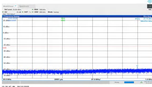
NTNV-n66-PC3-15-20-L-DFT-QPSK-Inner_1RB_Left-30-1000-PASS
