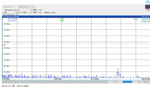
NTNV-n66-PC3-15-5-M-DFT-QPSK-Inner_1RB_Right-0.009-0.15 -PASS
