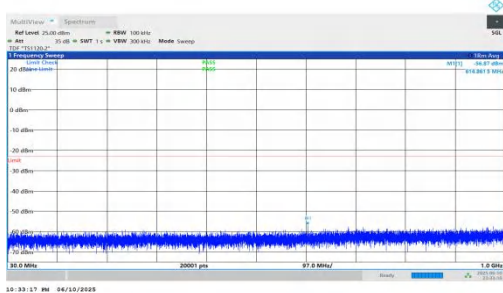
NTNV-n66-PC3-15-20-L-DFT-QPSK-Inner_1RB_Right-30-1000-P ASS
