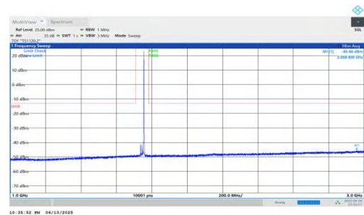
NTNV-n66-PC3-15-20-M-DFT-QPSK-Inner_1RB_Right-1000-3000-PASS
