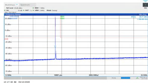
NTNV-n66-PC3-15-10-L-DFT-QPSK-Inner_1RB_Left-1000-3000-P ASS
