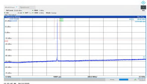
NTNV-n66-PC3-15-10-M-DFT-QPSK-Inner_1RB_Right-1000-3000- -PASS
