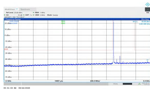
NTNV-n41-PC1.5-30-90-L-DFT-QPSK-Inner_1RB_Left-1000-3000 -PASS
