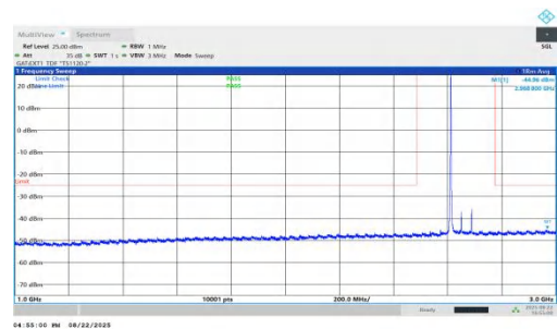
NTNV-n41-PC1.5-30-80-H-DFT-QPSK-Inner_1RB_Left-1000-3000 -PASS
