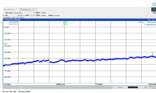
NTVN-n41-PC1.5-30-90-M-DFT-BPSK-Inner_1RB_Left-3000-180 00-PASS
