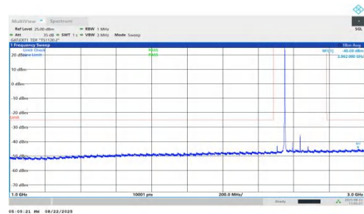
NTVN-n41-PC1.5-30-90-M-DFT-BPSK-Inner_1RB_Left-1000-3000 -PASS
