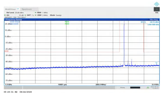
NTVN-n41-PC1.5-30-100-M-DFT-QPSK-Inner_1RB_Left-1000-30 00-PASS
