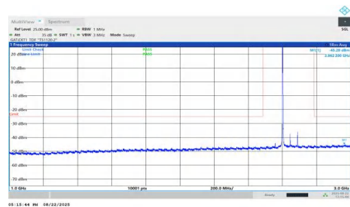
NTNV-n41-PC1.5-30-90-H-DFT-QPSK-Inner_1RB_Left-1000-3000 -PASS
