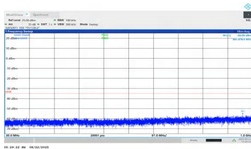
NTVN-n41-PC1.5-30-100-M-DFT-QPSK-Inner_1RB_Left-30-1000 -PASS
