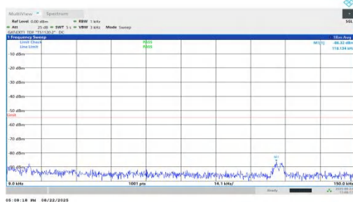
NTNV-n41-PC1.5-30-90-M-DFT-QPSK-Inner_1RB_Left-0.009-0.15-PASS
