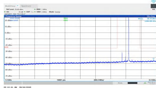
NTVN-n41-PC1.5-30-90-M-DFT-QPSK-Inner_1RB_Right-1000-3000-PASS
