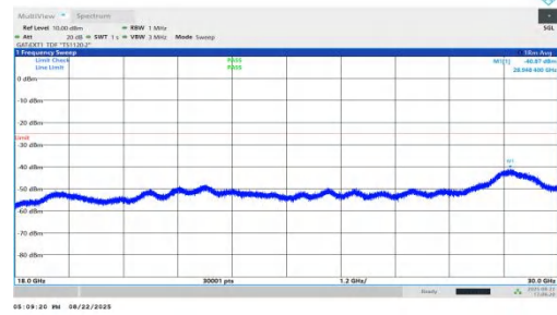
NTVN-n41-PC1.5-30-90-M-DFT-QPSK-Inner_1RB_Left-18000-30000-PASS
