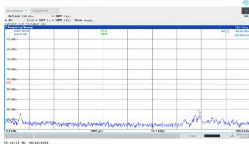
NTNV-n41-PC1.5-30-100-H-DFT-QPSK-Inner_1RB_Left-0.009-0. 15-PASS
