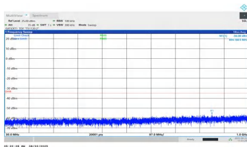
NTNV-n41-PC1.5-30-100-L-DFT-QPSK-Inner_1RB_Left-30-1000 -PASS
