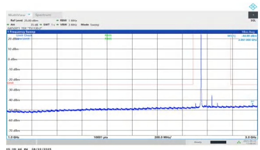
NTNV-n41-PC1.5-30-90-M-DFT-QPSK-Inner_1RB_Left-1000-3000-PASS
