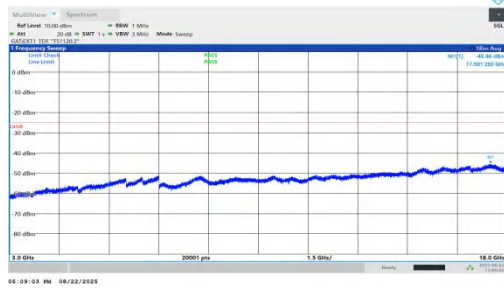
NTVN-n41-PC1.5-30-90-M-DFT-QPSK-Inner_1RB_Left-3000-18000-PASS
