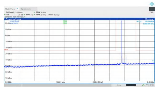
NTVN-n41-PC1.5-30-60-M-DFT-QPSK-Inner_1RB_Left-1000-300 0-PASS
