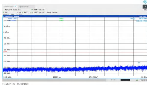
NTNV-n41-PC1.5-30-70-L-DFT-BPSK-Inner_1RB_Left-30-1000-P-ASS
