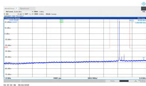
NTNV-n41-PC1.5-30-70-H-DFT-BPSK-Inner_1RB_Left-1000-3000 -PASS
