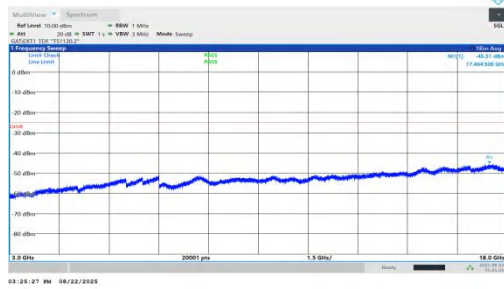
NTVN-n41-PC1.5-30-45-M-DFT-QPSK-Inner_1RB_Left-3000-18000-PASS
