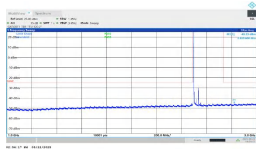
NTNV-n41-PC1.5-30-40-L-DFT-BPSK-Inner_1RB_Left-1000-3000 -PASS
