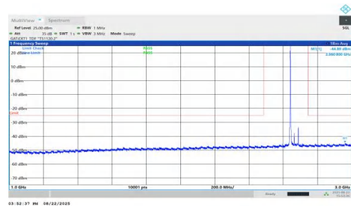
NTNV-n41-PC1.5-30-50-H-DFT-QPSK-Inner_1RB_Left-1000-3000 -PASS
