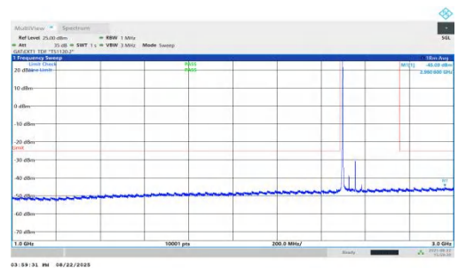
NTNV-n41-PC1.5-30-60-L-DFT-QPSK-Inner_1RB_Left-1000-3000 -PASS
