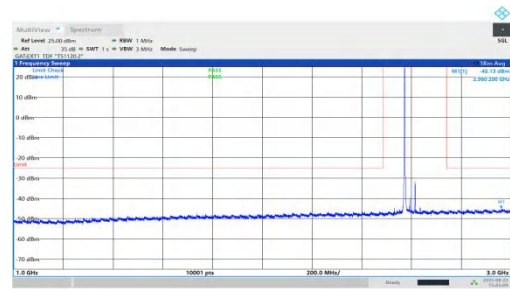
NTVN-n41-PC1.5-30-45-M-DFT-QPSK-Inner_1RB_Left-1000-3000-PASS
