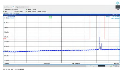
NTNV-n41-PC1.5-30-45-H-DFT-QPSK-Inner_1RB_Left-1000-3000 -PASS
