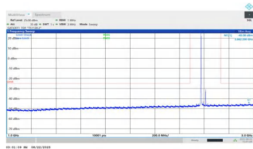
NTNV-n41-PC1.5-30-40-M-DFT-BPSK-Inner_1RB_Left-1000-3000 -PASS
