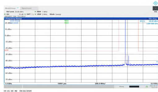
NTVN-n41-PC1.5-30-45-M-DFT-BPSK-Inner_1RB_Left-1000-3000 -PASS
