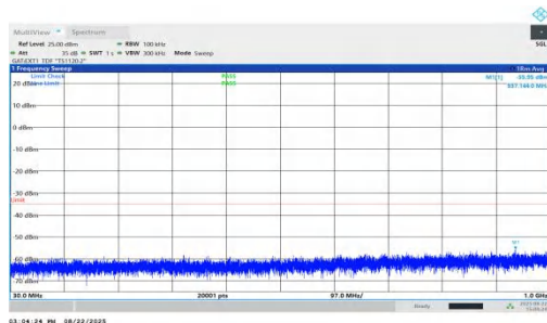
NTVN-n41-PC1.5-30-40-M-DFT-QPSK-Inner_1RB_Left-30-1000-PASS
