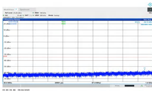
NTVN-n41-PC1.5-30-50-M-DFT-QPSK-Inner_1RB_Left-30-1000-PASS
