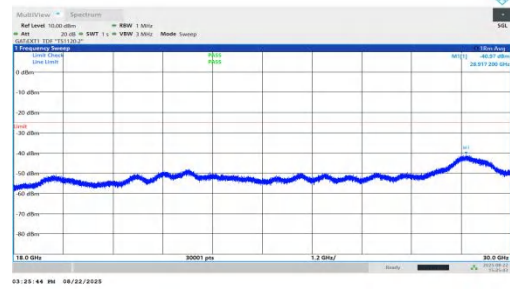
NTVN-n41-PC1.5-30-45-M-DFT-QPSK-Inner_1RB_Left-18000-30000-PASS
