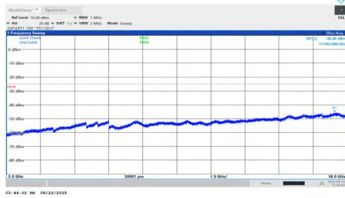
NTVN-n41-PC1.5-30-50-M-DFT-QPSK-Inner_1RB_Left-3000-18000-PASS
