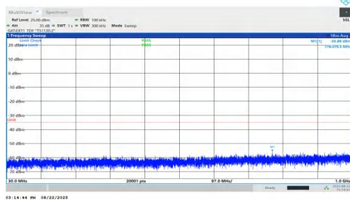
NTNV-n41-PC1.5-30-45-L-DFT-BPSK-Inner_1RB_Left-30-1000-P-ASS
