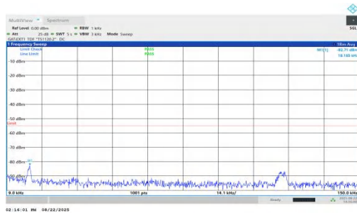
NTNV-n41-PC1.5-30-30-L-DFT-QPSK-Inner_1RB_Left-0.009-0.1 5-PASS
