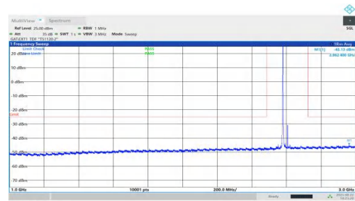
NTVN-n41-PC1.5-30-30-M-DFT-QPSK-Inner_1RB_Left-1000-3000-PASS
