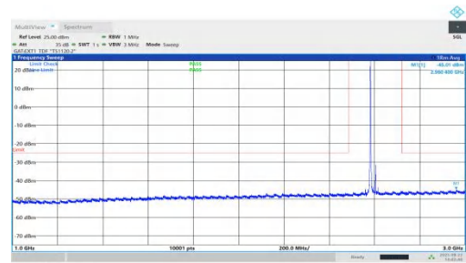
NTVN-n41-PC1.5-30-25-M-DFT-QPSK-Inner_1RB_Left-1000-3000-PASS
