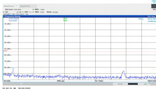
NTNV-n41-PC1.5-30-35-M-DFT-QPSK-Inner_1RB_Left-0.009-0.15-PASS
