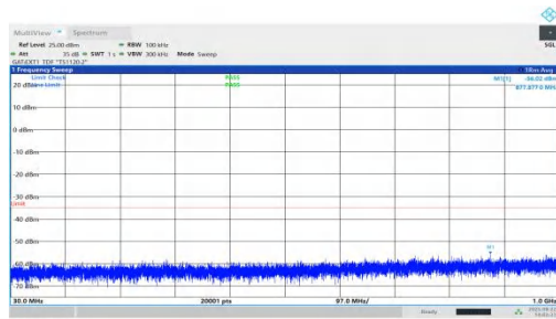
NTVN-n41-PC1.5-30-25-M-DFT-QPSK-Inner_1RB_Left-30-1000-PASS
