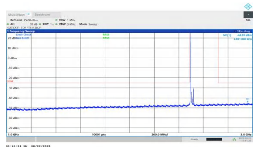
NTNV-n41-PC1.5-30-25-L-DFT-QPSK-Inner_1RB_Left-1000-3000 -PASS
