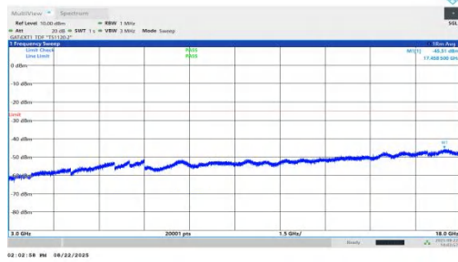
NTVN-n41-PC1.5-30-25-M-DFT-QPSK-Inner_1RB_Left-3000-18000-PASS
