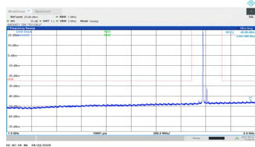
NTNV-n41-PC1.5-30-35-M-DFT-BPSK-Inner_1RB_Left-1000-3000 -PASS
