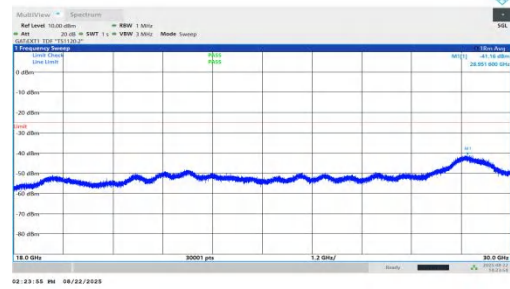
NTVN-n41-PC1.5-30-30-M-DFT-QPSK-Inner_1RB_Left-18000-3000-PASS
