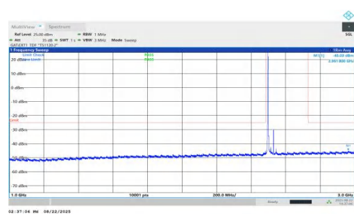
NTNV-n41-PC1.5-30-35-L-DFT-QPSK-Inner_1RB_Left-1000-3000 -PASS
