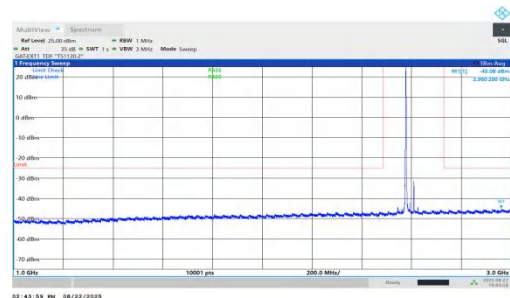
NTNV-n41-PC1.5-30-35-M-DFT-QPSK-Inner_1RB_Left-1000-3000-PASS
