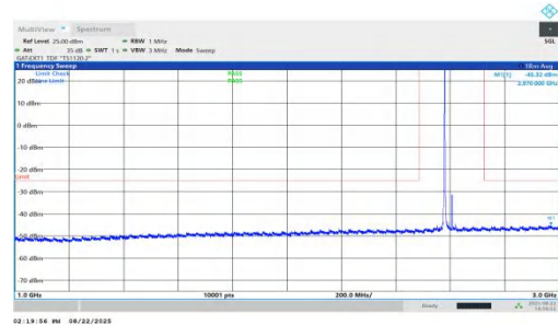
NTNV-n41-PC1.5-30-30-M-DFT-BPSK-Inner_1RB_Left-1000-3000 -PASS
