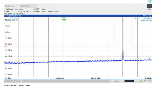
NTVN-n41-PC1.5-30-30-M-DFT-QPSK-Inner_1RB_Right-1000-3000-PASS
