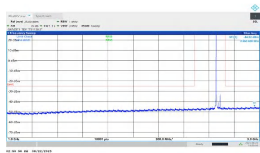
NTNV-n41-PC1.5-30-35-H-DFT-QPSK-Inner_1RB_Left-1000-3000 -PASS
