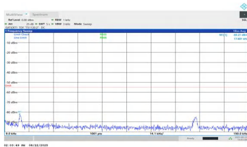
NTVN-n41-PC1.5-30-25-M-DFT-QPSK-Inner_1RB_Right-0.009-0.15-PASS
