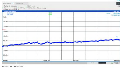
NTVN-n41-PC1.5-30-30-M-DFT-QPSK-Inner_1RB_Left-3000-18000-PASS
