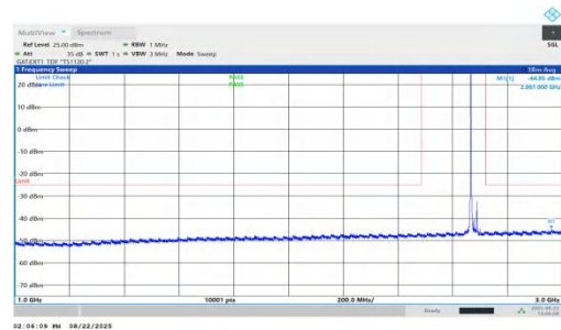
NTNV-n41-PC1.5-30-25-H-DFT-BPSK-Inner_1RB_Left-1000-3000 -PASS
