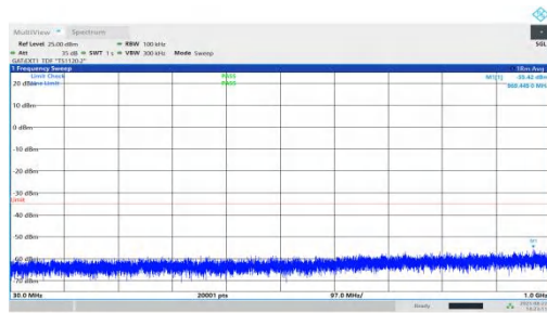
NTVN-n41-PC1.5-30-30-M-DFT-QPSK-Inner_1RB_Left-30-1000-PASS
