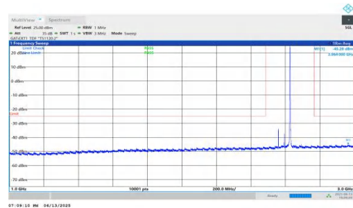
NTNV-n41-PC2-30-70-M-DFT-QPSK-Inner_1RB_Right-1000-3000- -PASS
