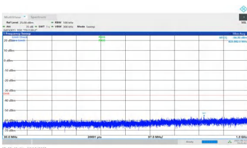
NTNV-n41-PC2-30-80-M-DFT-QPSK-Inner_1RB_Left-30-1000-PASS
