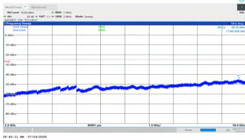
NTNV-n41-PC2-30-60-L-DFT-QPSK-Inner_1RB_Left-3000-18000 -PASS
