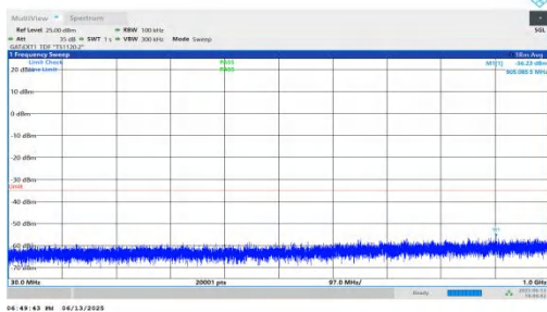
NTNV-n41-PC2-30-60-M-DFT-QPSK-Inner_1RB_Left-30-1000-PASS
