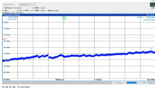
NTNV-n41-PC2-30-70-L-DFT-QPSK-Inner_1RB_Left-3000-18000 -PASS
