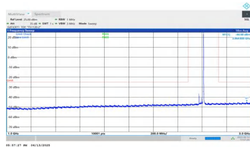
NTNV-n41-PC2-30-40-M-DFT-QPSK-Inner_1RB_Right-1000-3000- -PASS
