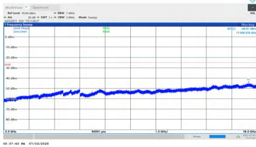
NTNV-n41-PC2-30-50-L-DFT-QPSK-Inner_1RB_Left-3000-18000 -PASS
