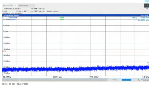
NTNV-n41-PC2-30-50-M-DFT-QPSK-Inner_1RB_Left-30-1000-PASS
