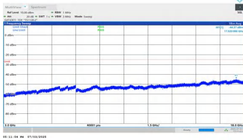
NTNV-n41-PC2-30-25-M-DFT-QPSK-Inner_1RB_Left-3000-1800 0-PASS
