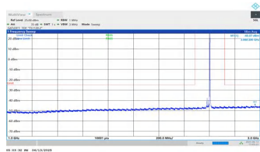
NTNV-n41-PC2-30-25-M-DFT-QPSK-Inner_1RB_Right-1000-3000- -PASS
