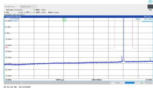
NTNV-n41-PC2-30-30-M-DFT-QPSK-Inner_1RB_Right-1000-3000- -PASS
