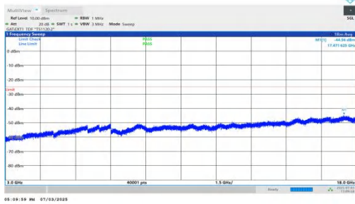
NTNV-n41-PC2-30-25-L-DFT-QPSK-Inner_1RB_Left-3000-18000 -PASS
