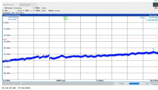
NTNV-n41-PC2-30-20-M-DFT-QPSK-Inner_1RB_Left-3000-1800 0-PASS
