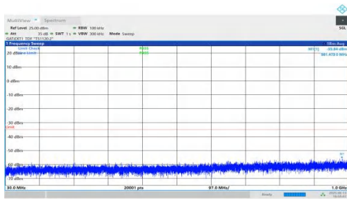
NTNV-n41-PC2-30-25-L-DFT-QPSK-Inner_1RB_Left-30-1000-PASS
