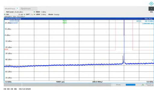
NTNV-n41-PC2-30-20-M-DFT-QPSK-Inner_1RB_Right-1000-3000- -PASS
