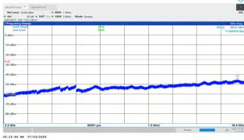
NTNV-n41-PC2-30-30-L-DFT-QPSK-Inner_1RB_Left-3000-18000 -PASS
