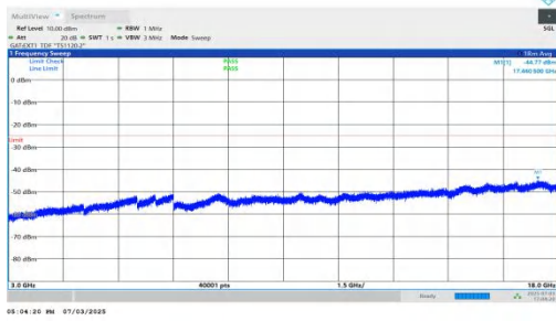
NTNV-n41-PC2-30-20-L-DFT-QPSK-Inner_1RB_Left-3000-18000 -PASS
