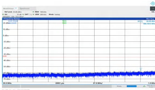
NTNV-n41-PC2-30-20-L-DFT-QPSK-Inner_1RB_Left-30-1000-PASS
