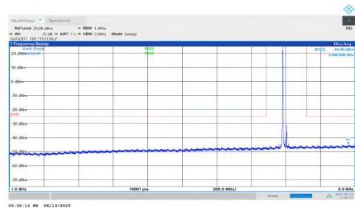
NTNV-n41-PC2-30-25-M-DFT-QPSK-Inner_1RB_Left-1000-3000-PASS
