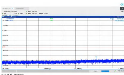
NTNV-n41-PC2-30-30-M-DFT-QPSK-Inner_1RB_Left-30-1000-PASS
