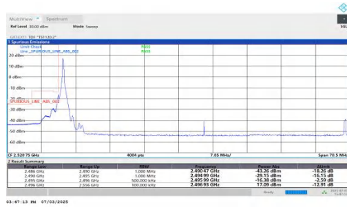
NTVN-n41-PC2-30-60-L-DFT-BPSK-Edge_1RB_Left-PASS
