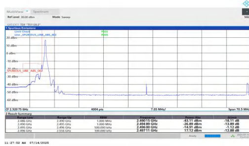
NTVN-n41-PC2-30-60-L-DFT-QPSK-Edge_1RB_Left-PASS
