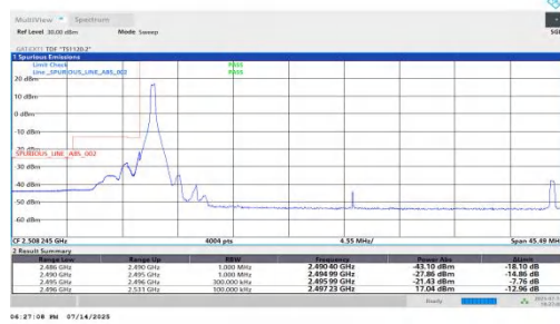
NTVN-n41-PC2-30-35-L-DFT-QPSK-Edge_1RB_Left-PASS
