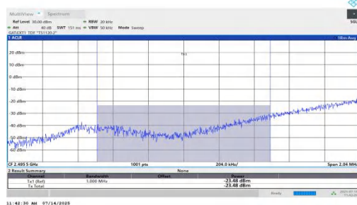
NTVN-n41-PC2-30-90-L-DFT-BPSK-Edge_1RB_Left-PASS
