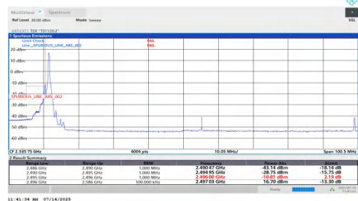
NTVN-n41-PC2-30-90-L-DFT-BPSK-Edge_1RB_Left
