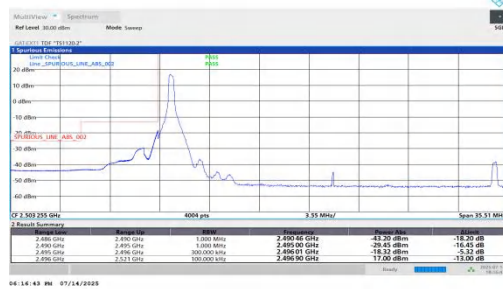
NTVN-n41-PC2-30-25-L-DFT-BPSK-Edge_1RB_Left-PASS
