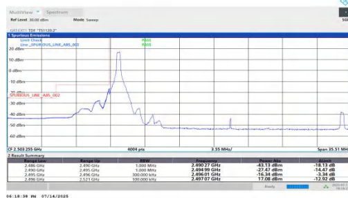
NTVN-n41-PC2-30-25-L-DFT-QPSK-Edge_1RB_Left-PASS
