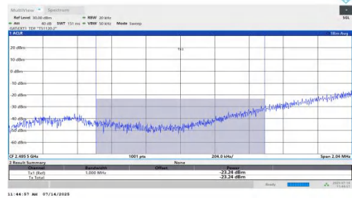
NTVN-n41-PC2-30-90-L-DFT-QPSK-Edge_1RB_Left-PASS
