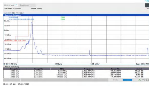
NTVN-n41-PC2-30-50-L-DFT-QPSK-Edge_1RB_Left-PASS
