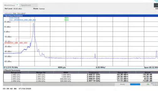
NTVN-n41-PC2-30-50-L-DFT-BPSK-Edge_1RB_Left-PASS
