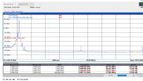
NTVN-n41-PC2-30-90-L-DFT-QPSK-Edge_1RB_Left
