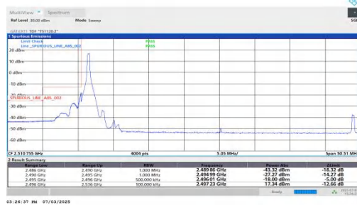
NTVN-n41-PC2-30-40-L-DFT-QPSK-Edge_1RB_Left-PASS
