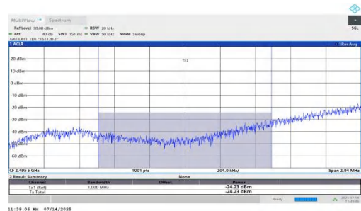
NTNV-n41-PC2-30-80-L-DFT-QPSK-Edge_1RB_Left-PASS
