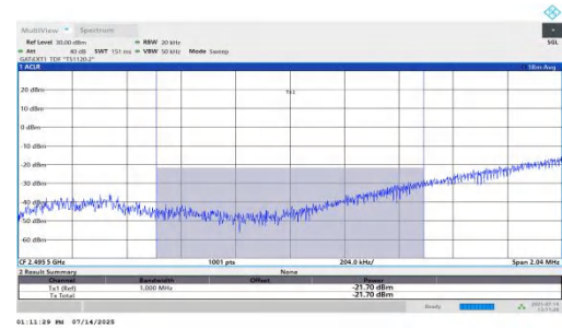
NTV-n41-PC2-30-100-L-DFT-QPSK-Edge_1RB_Left-PASS
