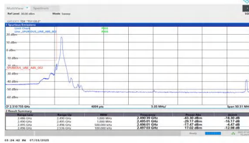
NTVN-n41-PC2-30-40-L-DFT-BPSK-Edge_1RB_Left-PASS
