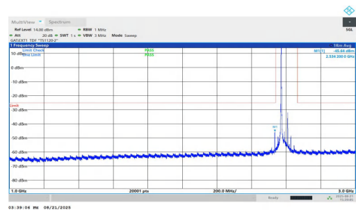
NTNV-n38-PC1.5-30-40-L-DFT-QPSK-Inner_1RB_Left-1000-3000 -PASS
