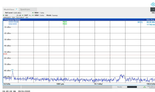
NTVN-n38-PC1.5-30-40-M-DFT-QPSK-Inner_1RB_Left-0.009-0.15-PASS
