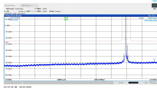
NTNV-n38-PC1.5-30-25-M-DFT-BPSK-Inner_1RB_Left-1000-3000 -PASS
