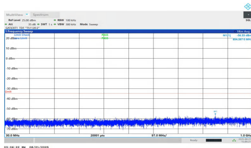
NTVN-n38-PC1.5-30-25-M-DFT-QPSK-Inner_1RB_Left-30-1000-PASS
