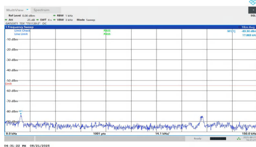
NTVN-n38-PC1.5-30-25-M-DFT-QPSK-Inner_1RB_Left-0.009-0.15-PASS
