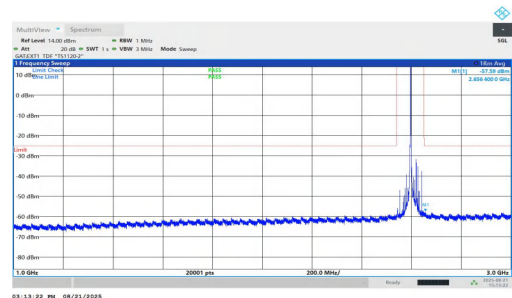
NTVN-n38-PC1.5-30-25-H-DFT-QPSK-Inner_1RB_Left-1000-3000 -PASS
