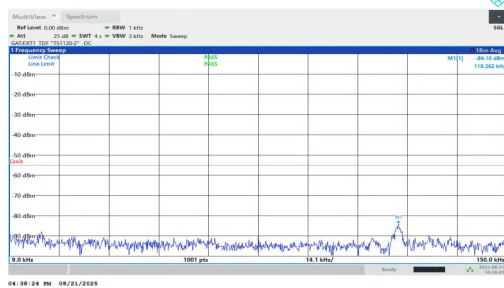
NTVN-n38-PC1.5-30-30-M-DFT-QPSK-Inner_1RB_Left-0.009-0.15-PASS
