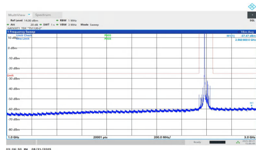
NTVN-n38-PC1.5-30-25-M-DFT-QPSK-Inner_1RB_Left-1000-3000-PASS
