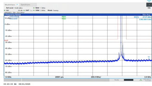
NTNV-n38-PC1.5-30-30-M-DFT-BPSK-Inner_1RB_Left-1000-3000 -PASS
