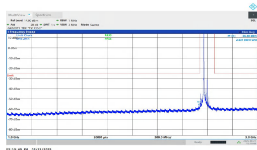
NTNV-n38-PC1.5-30-30-L-DFT-QPSK-Inner_1RB_Left-1000-3000 -PASS
