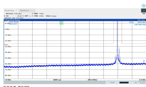
NTVN-n38-PC1.5-30-30-H-DFT-QPSK-Inner_1RB_Left-1000-3000 -PASS
