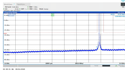
NTNV-n38-PC1.5-30-20-L-DFT-BPSK-Inner_1RB_Left-1000-3000 -PASS
