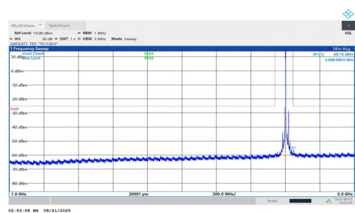
NTVN-n38-PC1.5-30-20-H-DFT-QPSK-Inner_1RB_Left-1000-3000 -PASS
