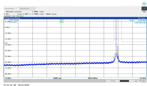
NTNV-n38-PC1.5-30-25-L-DFT-QPSK-Inner_1RB_Left-1000-3000 -PASS
