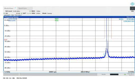
NTNV-n38-PC1.5-30-20-L-DFT-QPSK-Inner_1RB_Left-1000-3000 -PASS
