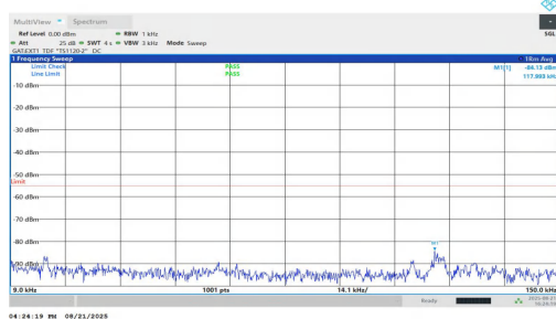
NTVN-n38-PC1.5-30-20-M-DFT-QPSK-Inner_1RB_Left-0.009-0.15-PASS
