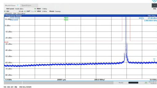
NTNV-n38-PC1.5-30-20-M-DFT-BPSK-Inner_1RB_Left-1000-3000 -PASS
