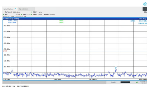
NTVN-n38-PC1.5-30-10-M-DFT-QPSK-Inner_1RB_Left-0.009-0.15-PASS
