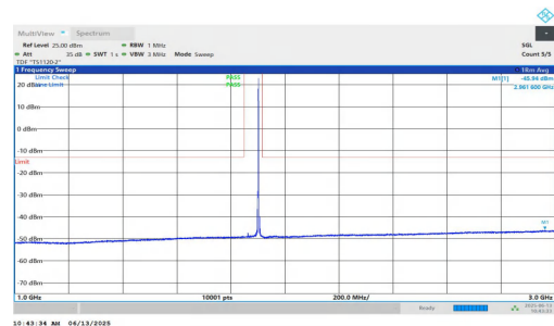
NTNV-n25-PC3-15-40-M-DFT-QPSK-Inner_1RB_Right-1000-3000- -PASS
