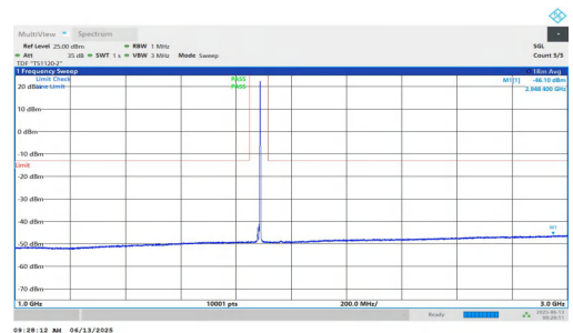
NTNV-n25-PC3-15-10-M-DFT-QPSK-Inner_1RB_Right-1000-3000 -PASS
