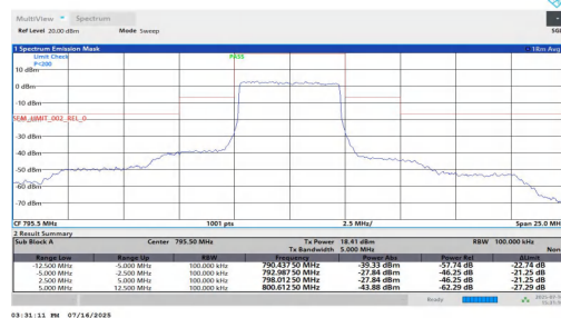
NTNT-n14-PC3-15-5-H-DFT-QPSK-Outer Full--5.00--2.50-PASS
