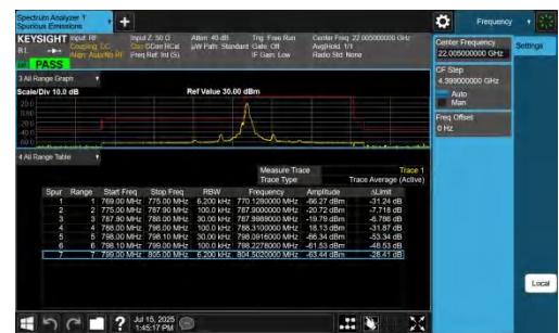
NTNV-n14-PC3-15-5-L-DFT-QPSK-Edge_1RB_Left-PASS
