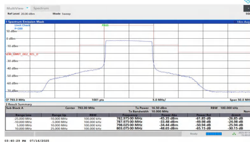
NTNT-n14-PC3-15-10-L-CP-QPSK-Outer_Full--10.00--5.00-PAS
