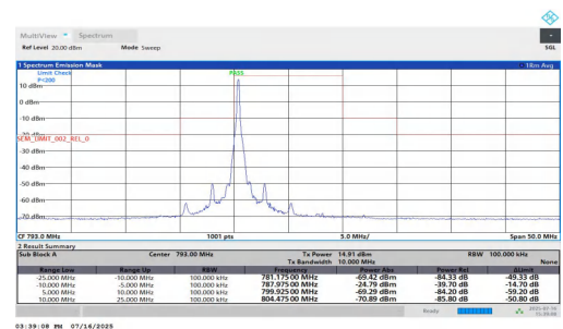
NTNT-n14-PC3-15-10-L-DFT-64QAM-Edge_1RB_Left--10.00--5. 00-PASS
