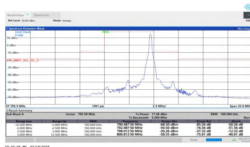
NTNT-n14-PC3-15-5-H-DFT-16QAM-Edge_1RB_Right--5.00--2.5 0-PASS
