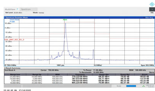
NTNT-n14-PC3-15-10-L-CP-256QAM-Edge_1RB_Left--10.00--5.00-PASS
