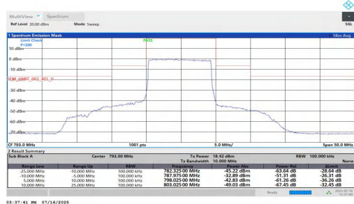
NTNT-n14-PC3-15-10-L-DFT-QPSK-Outer_Full--10.00--5.00-PAS
