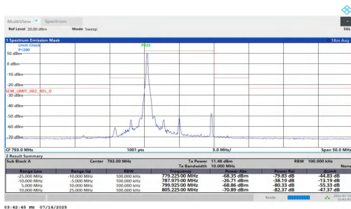
NTNT-n14-PC3-15-10-L-CP-256QAM-Edge_1RB_Left--25.00--10.00-PASS
