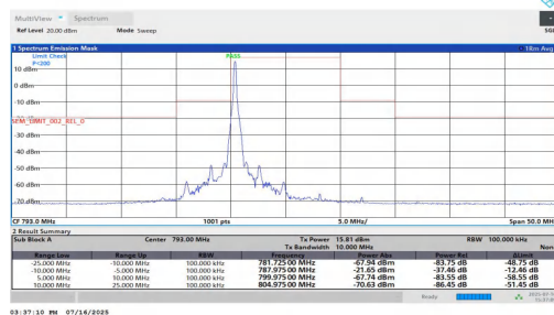
NTNT-n14-PC3-15-10-L-DFT-BPSK-Edge_1RB_Left--10.00--5.00 -PASS
