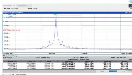
NTNT-n14-PC3-15-10-L-CP-64QAM-Edge_1RB_Left--10.00--5.0 0-PASS
