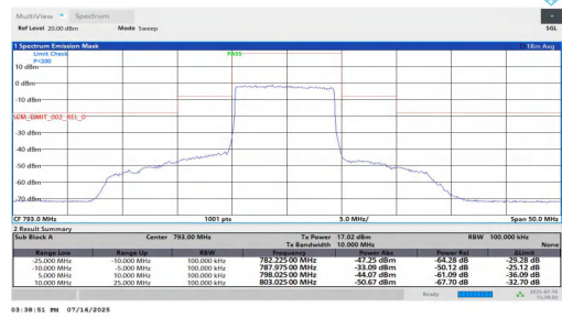
NTNT-n14-PC3-15-10-L-DFT-64QAM-Outer_Full--10.00--5.00-PA SS
