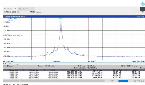
NTNT-n14-PC3-15-10-L-DFT-16QAM-Edge_1RB_Left--10.00--5. 00-PASS
