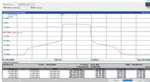
NTNT-n14-PC3-15-10-L-CP-64QAM-Out_Full--25.00--10.00-PA SS
