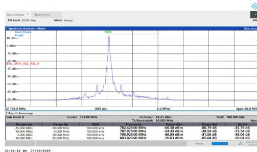
NTNT-n14-PC3-15-10-L-CP-16QAM-Edge_1RB_Left--10.00--5.0
