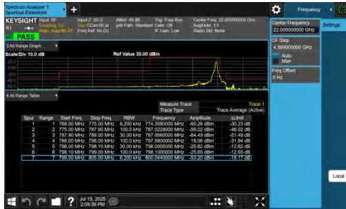
NTNV-n14-PC3-15-10-L-DFT-QPSK-Edge_1RB_Right-PASS
