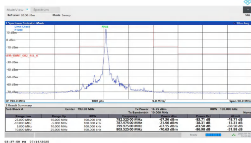
NTNT-n14-PC3-15-10-L-DFT-QPSK-Edge_1RB_Left--10.00--5.0 0-PASS
