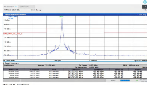
NTNT-n14-PC3-15-10-L-DFT-QPSK-Edge_1RB_Left-10.00-25.00 -PASS
