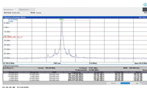
NTNT-n14-PC3-15-10-L-DFT-64QAM-Edge_1RB_Left--25.00--10.00-PASS
