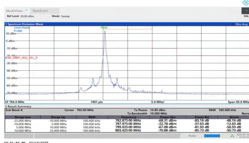
NTNT-n14-PC3-15-10-L-CP-64QAM-Edge_1RB_Left--25.00--10.0 0-PASS
