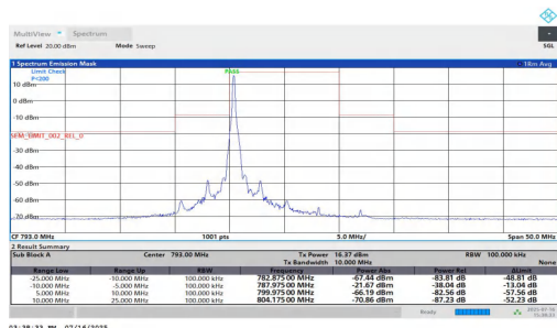
NTNT-n14-PC3-15-10-L-DFT-16QAM-Edge_1RB_Left--25.00--10. 00-PASS
