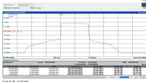
NTNT-n14-PC3-15-10-L-CP-QPSK-Outer_Full--25.00--10.00-PAS
