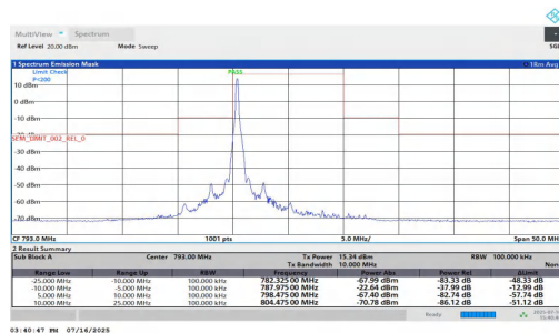
NTNT-n14-PC3-15-10-L-CP-QPSK-Edge_1RB_Left--10.00--5.00-
