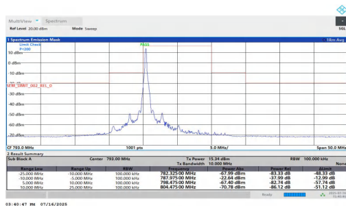
NTNT-n14-PC3-15-10-L-CP-QPSK-Edge_1RB_Left--25.00--10.00
