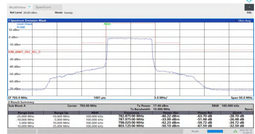
NTNT-n14-PC3-15-10-L-DFT-16QAM-Outer_Full--10.00--5.00-PA SS
