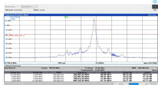
NTNT-n14-PC3-15-5-H-CP-64QAM-Edge_1RB_Right--5.00--2.50 -PASS
