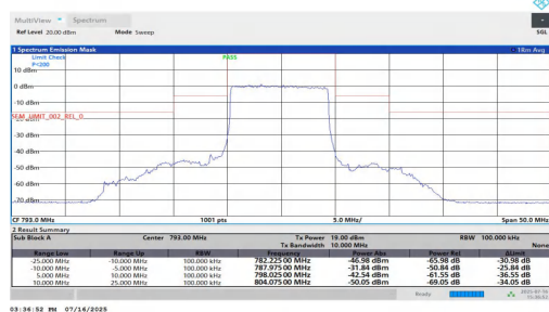
NTNT-n14-PC3-15-10-L-DFT-BPSK-Outer_Full--10.00--5.00-PAS
