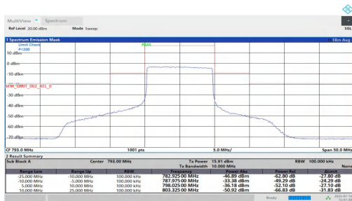
NTNT-n14-PC3-15-10-L-CP-64QAM-Out_Full--25.00--10.00-PA SS
