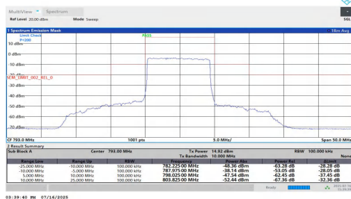
NTNT-n14-PC3-15-10-L-DFT-256QAM-Outer_Full--25.00--10.00-P
