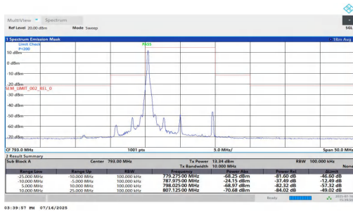
NTNT-n14-PC3-15-10-L-DFT-256QAM-Edge_1RB_Left--25.00--10.00-PASS
