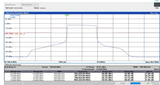
NTNT-n14-PC3-15-10-L-CP-64QAM-Out_Full--10.00--5.00-PA SS
