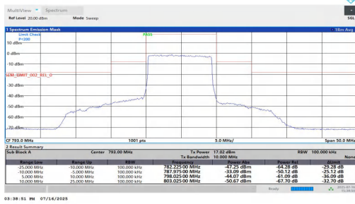
NTNT-n14-PC3-15-10-L-DFT-64QAM-Outer_Full--25.00--10.00-PA SS
