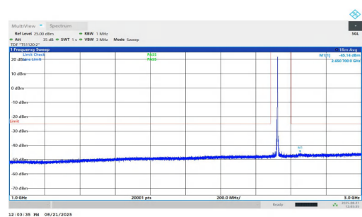
NTNV-n7-PC2-15-25-M-DFT-QPSK-Inner_1RB_Left-1000-3000-P ASS
