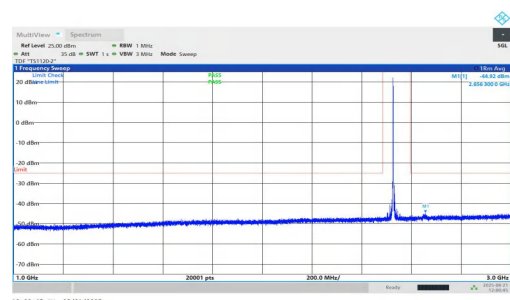
NTNV-n7-PC2-15-20-M-DFT-QPSK-Inner_1RB_Left-1000-3000-P ASS
