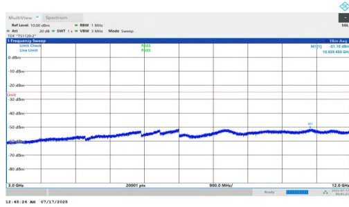
NTNV-n7-PC2-15-20-M-DFT-QPSK-Inner_1RB_Left-3000-12000 -PASS
