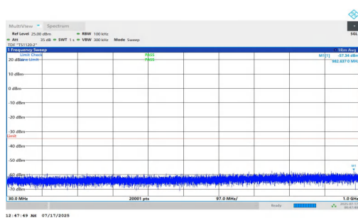
NTNV-n7-PC2-15-20-H-DFT-QPSK-Inner_1RB_Left-30-1000-P ASS
