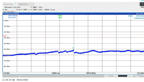
NTNV-n7-PC2-15-25-M-DFT-QPSK-Inner_1RB_Left-3000-12000 -PASS
