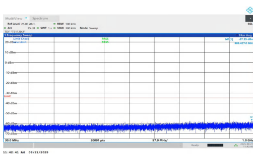
NTNV-n7-PC2-15-25-H-DFT-QPSK-Inner_1RB_Left-30-1000-P ASS
