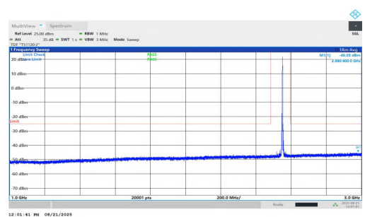
NTNV-n7-PC2-15-20-H-DFT-QPSK-Inner_1RB_Left-1000-3000-P ASS
