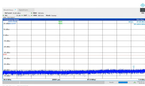
NTNV-n7-PC2-15-20-M-DFT-QPSK-Inner_1RB_Left-30-1000-PA SS
