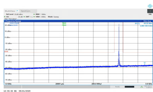
NTNV-n7-PC2-15-25-H-DFT-QPSK-Inner_1RB_Left-1000-3000-P ASS
