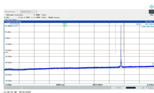
NTNV-n7-PC2-15-15-H-DFT-QPSK-Inner_1RB_Left-1000-3000-P ASS
