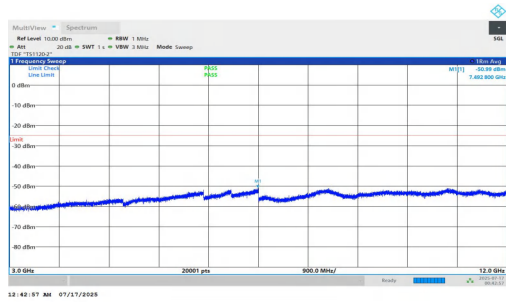
NTNV-n7-PC2-15-20-L-DFT-QPSK-Inner_1RB_Left-3000-12000-PASS
