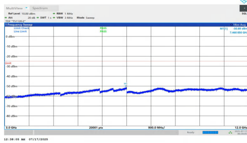
NTNV-n7-PC2-15-15-M-DFT-QPSK-Inner_1RB_Left-3000-12000 -PASS
