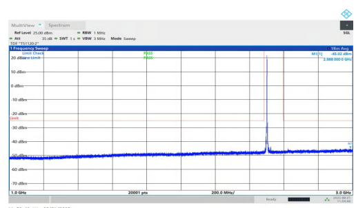
NTNV-n7-PC2-15-20-L-DFT-QPSK-Inner_1RB_Left-1000-3000-PA SS
