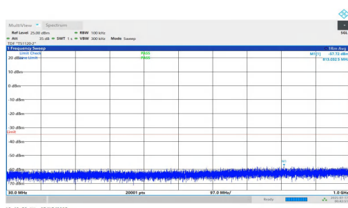
NTNV-n7-PC2-15-20-L-DFT-QPSK-Inner_1RB_Left-30-1000-PA SS
