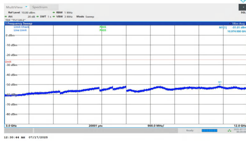
NTNV-n7-PC2-15-10-M-DFT-QPSK-Inner_1RB_Left-3000-12000 -PASS
