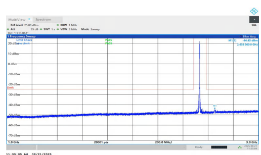
NTNV-n7-PC2-15-10-M-DFT-QPSK-Inner_1RB_Left-1000-3000-P ASS
