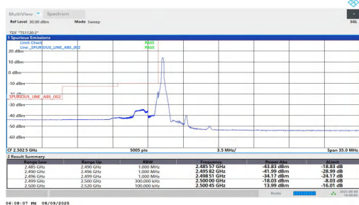
NTNV-n7-PC2-15-15-L-DFT-QPSK-Edge 1RB Left-PASS
