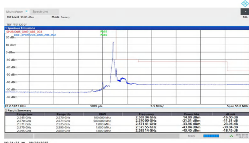
NTNV-n7-PC2-15-25-H-DFT-QPSK-Edge 1RB Right-PASS
