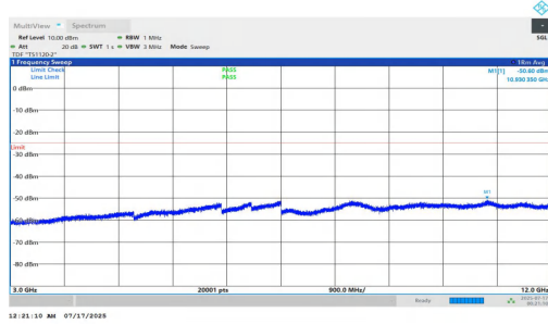
NTNV-n7-PC2-15-5-L-DFT-QPSK-Inner_1RB_Left-3000-12000-P ASS
