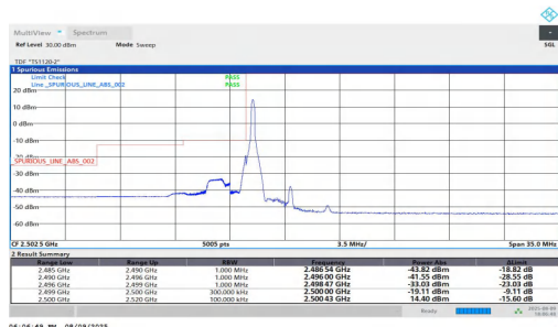
NTNV-n7-PC2-15-15-L-DFT-BPSK-Edge 1RB Left-PASS
