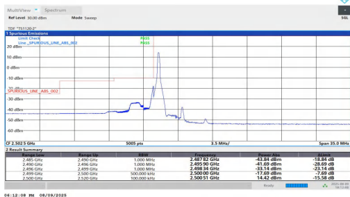
NTNV-n7-PC2-15-20-L-DFT-BPSK-Edge_1RB_Left-PASS
