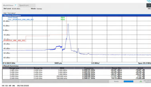
NTNV-n7-PC2-15-10-L-DFT-QPSK-Edge_1RB_Left-PASS
