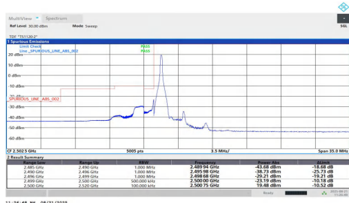
NTNV-n7-PC2-15-50-L-DFT-QPSK-Edge 1RB Left-PASS
