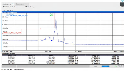
NTNV-n7-PC2-15-10-L-DFT-BPSK-Edge_1RB_Left-PASS
