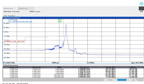
NTNV-n7-PC2-15-30-L-DFT-BPSK-Edge 1RB Left-PASS
