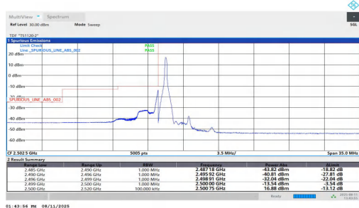
NTNV-n7-PC2-15-50-L-DFT-BPSK-Edge 1RB Left-PASS
