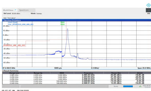
NTNV-n7-PC2-15-5-L-DFT-QPSK-Edge 1RB Left-PASS
