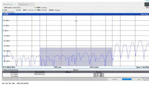
NTNV-n7-PC2-15-40-L-DFT-QPSK-Edge_1RB_Left-PASS
