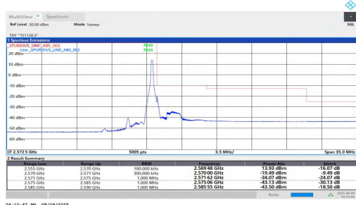
NTNV-n7-PC2-15-15-H-DFT-QPSK-Edge 1RB Right-PASS
