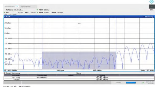
NTNV-n7-PC2-15-40-L-DFT-BPSK-Edge 1RB Left-PASS
