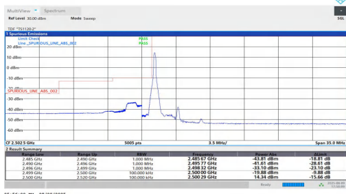
NTNV-n7-PC2-15-5-L-DFT-BPSK-Edge 1RB Left-PASS
