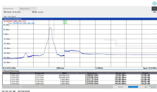
NTNV-n7-PC2-15-5-H-DFT-QPSK-Edge 1RB Right-PASS
