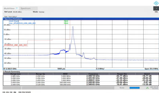
NTNV-n7-PC2-15-30-L-DFT-QPSK-Edge 1RB Left-PASS
