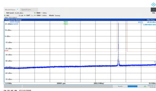
NTNV-n7-PC3-15-40-L-DFT-QPSK-Inner_1RB_Left-1000-3000-PA SS
