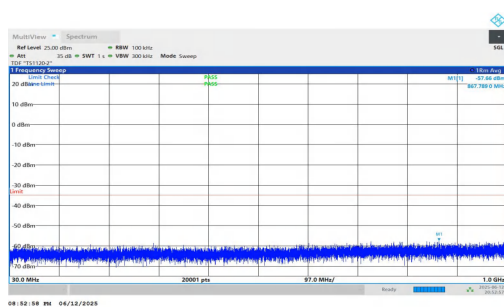
NTNV-n7-PC3-15-40-H-DFT-QPSK-Inner_1RB_Left-30-1000-P ASS
