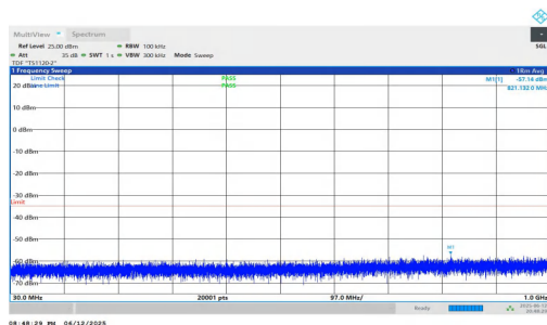
NTNV-n7-PC3-15-40-L-DFT-QPSK-Inner_1RB_Left-30-1000-PA SS
