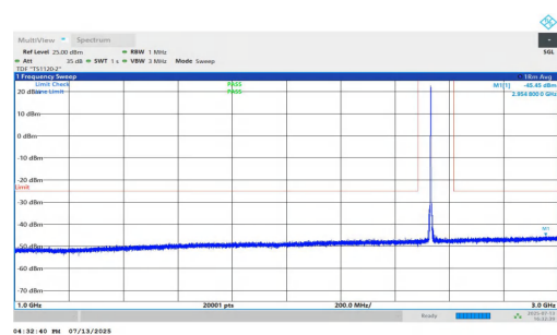
NTNV-n7-PC3-15-40-H-DFT-QPSK-Inner_1RB_Left-1000-3000-P ASS
