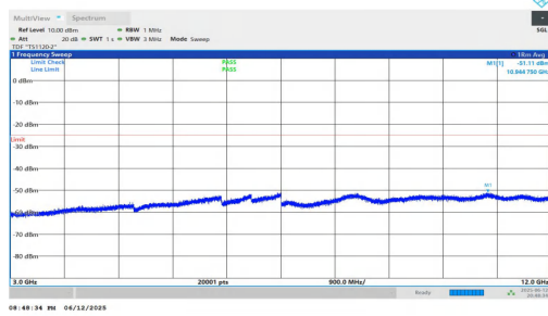
NTNV-n7-PC3-15-40-L-DFT-QPSK-Inner_1RB_Left-3000-12000-PASS
