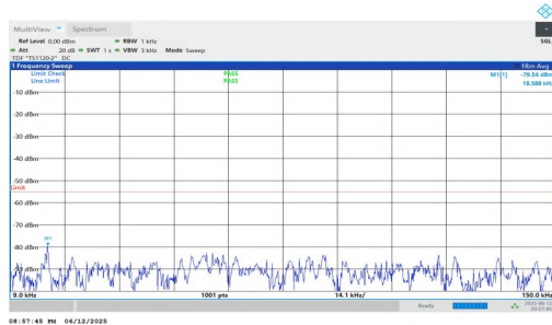
NTNV-n7-PC3-15-50-M-DFT-QPSK-Inner_1RB_Right-0.009-0.15 -PASS
