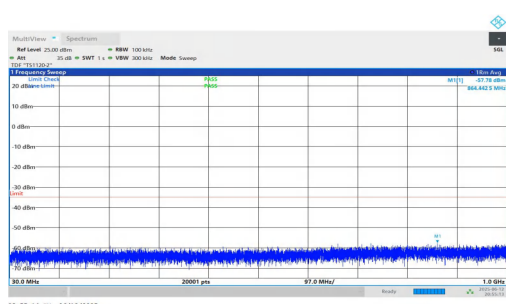
NTNV-n7-PC3-15-50-L-DFT-QPSK-Inner_1RB_Left-30-1000-PA SS
