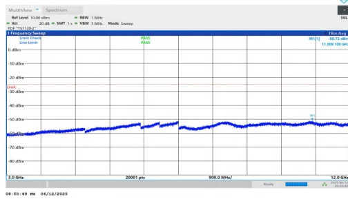
NTNV-n7-PC3-15-40-M-DFT-QPSK-Inner_1RB_Left-3000-12000 -PASS
