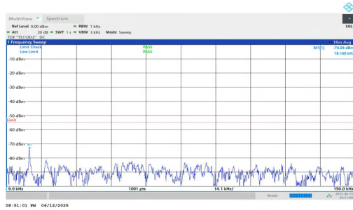
NTNV-n7-PC3-15-40-M-DFT-QPSK-Inner_1RB_Right-0.009-0.15 -PASS
