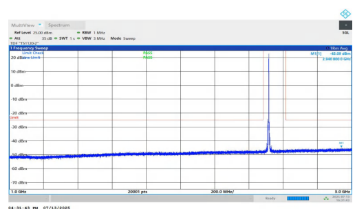
NTNV-n7-PC3-15-40-M-DFT-QPSK-Inner_1RB_Left-1000-3000-P ASS
