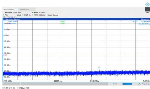
NTNV-n7-PC3-15-50-M-DFT-QPSK-Inner_1RB_Left-30-1000-PA SS
