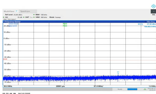
NTNV-n7-PC3-15-40-M-DFT-QPSK-Inner_1RB_Left-30-1000-PA SS
