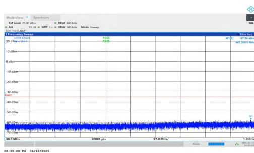
NTNV-n7-PC3-15-30-H-DFT-QPSK-Inner_1RB_Left-30-1000-P ASS
