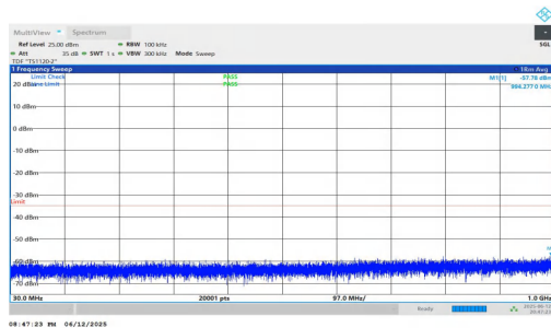
NTNV-n7-PC3-15-40-L-DFT-BPSK-Inner_1RB_Left-30-1000-PAS S
