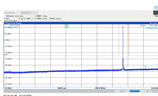
NTNV-n7-PC3-15-35-H-DFT-QPSK-Inner_1RB_Left-1000-3000-P ASS
