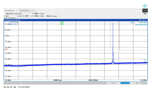
NTNV-n7-PC3-15-35-M-DFT-QPSK-Inner_1RB_Left-1000-3000-P ASS
