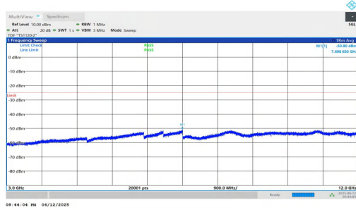
NTNV-n7-PC3-15-35-M-DFT-QPSK-Inner_1RB_Left-3000-12000 -PASS
