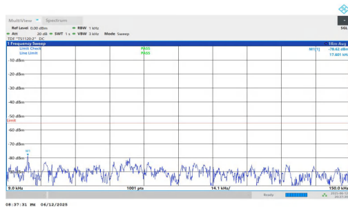
NTNV-n7-PC3-15-30-M-DFT-QPSK-Inner_1RB_Right-0.009-0.15 -PASS
