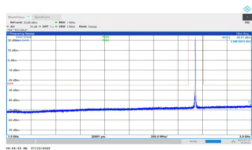
NTNV-n7-PC3-15-30-H-DFT-QPSK-Inner_1RB_Left-1000-3000-P ASS
