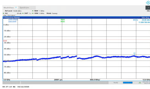
NTNV-n7-PC3-15-30-M-DFT-QPSK-Inner_1RB_Left-3000-12000 -PASS
