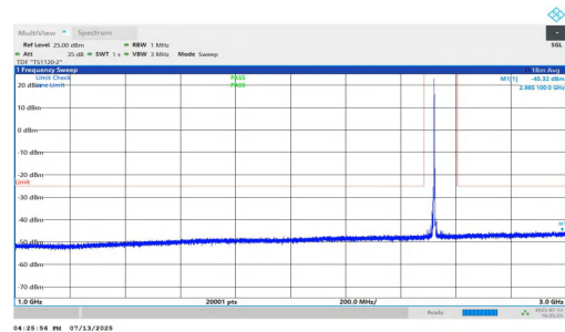
NTNV-n7-PC3-15-30-M-DFT-QPSK-Inner_1RB_Left-1000-3000-P ASS
