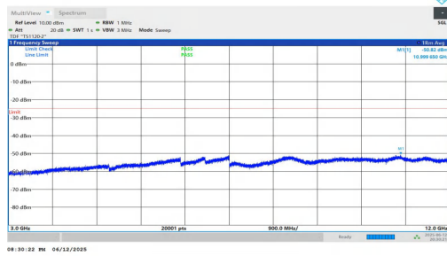
NTNV-n7-PC3-15-25-M-DFT-QPSK-Inner_1RB_Left-3000-12000 -PASS
