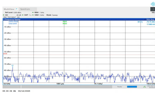
NTNV-n7-PC3-15-25-M-DFT-QPSK-Inner_1RB_Right-0.009-0.15 -PASS
