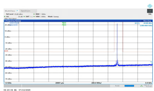
NTNV-n7-PC3-15-25-M-DFT-QPSK-Inner_1RB_Left-1000-3000-P ASS
