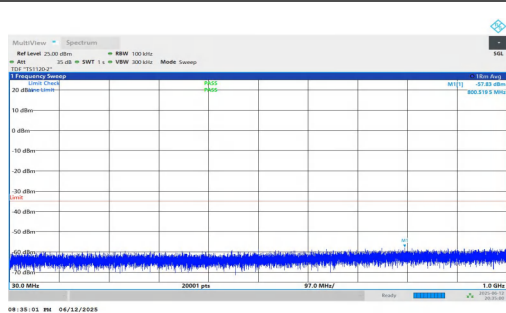
NTNV-n7-PC3-15-30-L-DFT-QPSK-Inner_1RB_Left-30-1000-PA SS
