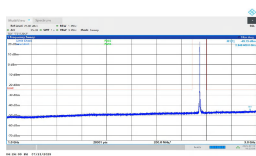
NTNV-n7-PC3-15-25-H-DFT-QPSK-Inner_1RB_Left-1000-3000-P ASS
