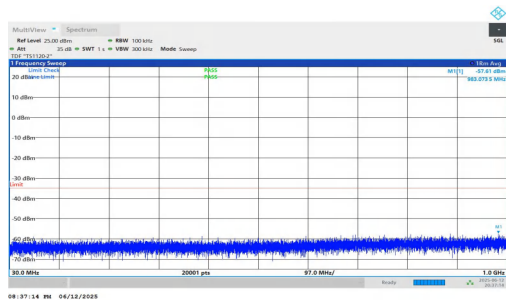
NTNV-n7-PC3-15-30-M-DFT-QPSK-Inner_1RB_Left-30-1000-PA SS
