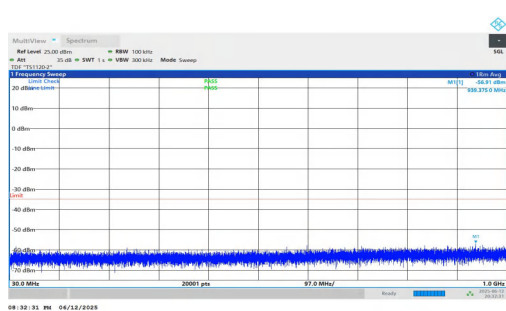
NTNV-n7-PC3-15-25-H-DFT-QPSK-Inner_1RB_Left-30-1000-P ASS
