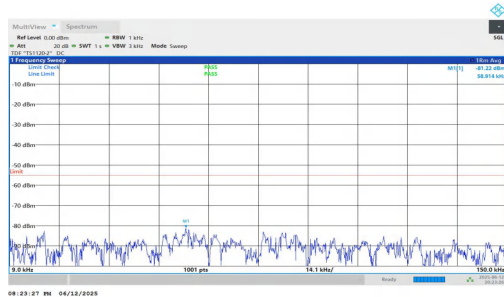
NTNV-n7-PC3-15-20-M-DFT-QPSK-Inner_1RB_Right-0.009-0.15 -PASS
