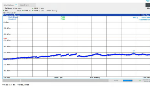
NTNV-n7-PC3-15-20-M-DFT-QPSK-Inner_1RB_Left-3000-12000 -PASS
