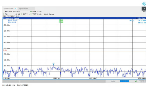
NTVN-n7-PC3-15-15-H-DFT-QPSK-Inner_1RB_Right-0.009-0.15 -PASS
