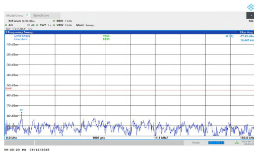
NTNV-n7-PC3-15-20-L-DFT-QPSK-Inner_1RB_Left-0.009-0.15-P ASS
