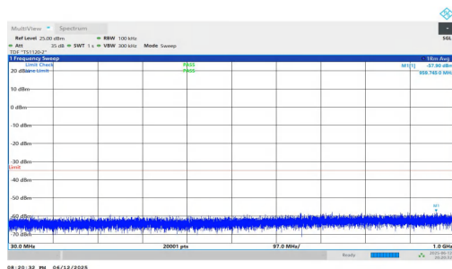
NTNV-n7-PC3-15-20-L-DFT-QPSK-Inner_1RB_Left-30-1000-PA SS
