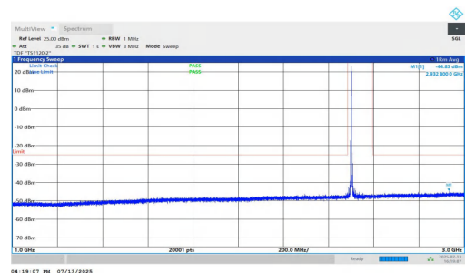
NTNV-n7-PC3-15-20-L-DFT-QPSK-Inner_1RB_Left-1000-3000-PA SS
