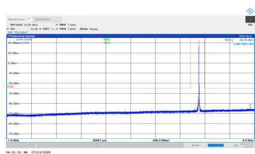
NTNV-n7-PC3-15-20-H-DFT-QPSK-Inner_1RB_Left-1000-3000-P ASS
