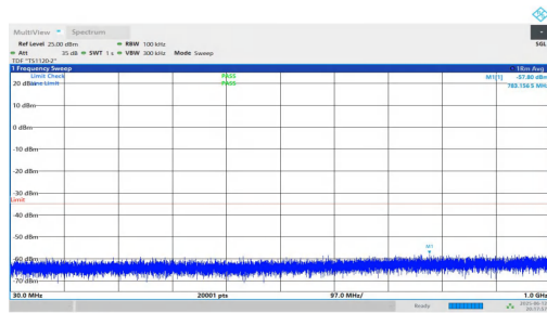
NTNV-n7-PC3-15-15-H-DFT-QPSK-Inner_1RB_Left-30-1000-P ASS
