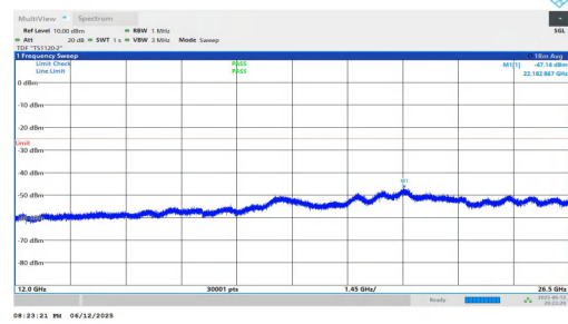
NTNV-n7-PC3-15-20-M-DFT-QPSK-Inner_1RB_Left-12000-26500 -PASS
