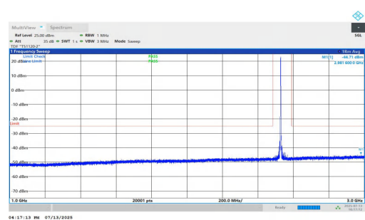
NTNV-n7-PC3-15-15-M-DFT-QPSK-Inner_1RB_Left-1000-3000-P ASS
