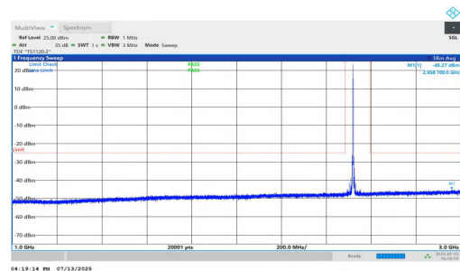
NTNV-n7-PC3-15-20-L-DFT-QPSK-Inner_1RB_Right-1000-3000-PASS
