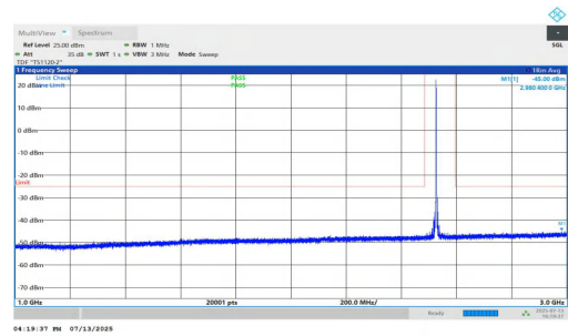
NTNV-n7-PC3-15-20-M-DFT-BPSK-Inner_1RB_Left-1000-3000-P ASS
