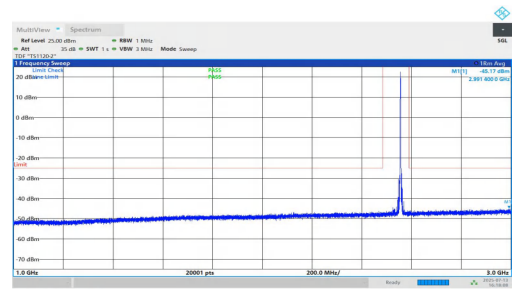
NTNV-n7-PC3-15-15-H-DFT-QPSK-Inner_1RB_Left-1000-3000-P ASS
