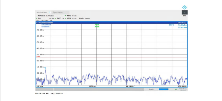
NTNV-n7-PC3-15-10-M-DFT-QPSK-Inner_1RB_Right-0.009-0.15 -PASS
