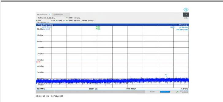
NTNV-n7-PC3-15-10-H-DFT-QPSK-Inner_1RB_Left-30-1000-P ASS
