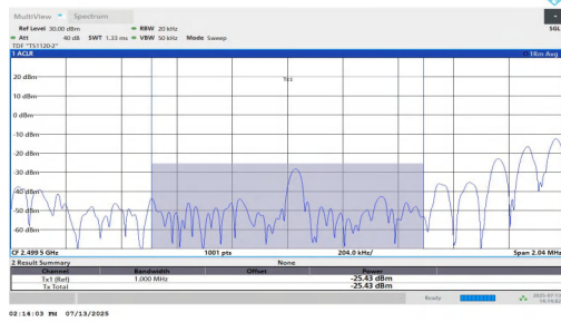
NTNV-n7-PC3-15-50-L-DFT-QPSK-Edge_1RB_Left-PASS
