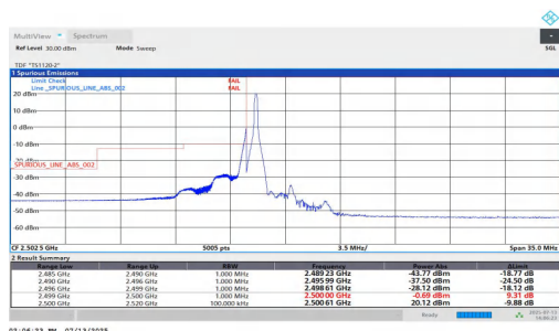
NTNV-n7-PC3-15-40-L-DFT-BPSK-Edge 1RB Left
