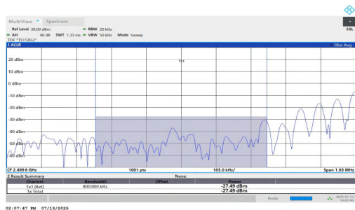
NTNV-n7-PC3-15-40-L-DFT-QPSK-Edge 1RB Left-PASS
