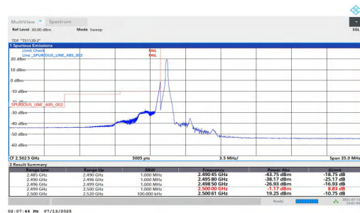
NTNV-n7-PC3-15-40-L-DFT-QPSK-Edge 1RB Left
