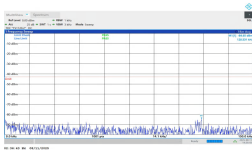
NTNV-n2-PC3-15-20-M-DFT-QPSK-Inner_1RB_Right-0.009-0.15 -PASS
