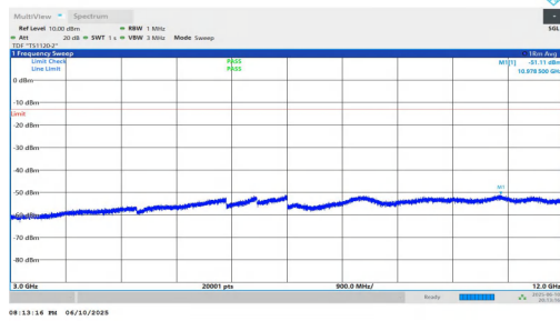
NTNV-n2-PC3-15-20-M-DFT-QPSK-Inner_1RB_Left-3000-12000 -PASS
