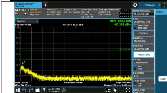
66-66-10MHz-20MHz-QPSK-QPSK-132328-132472-1RB#0-0RB #0-0.15~30MHz-PASS
