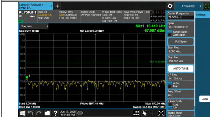
66-66-5MHz-20MHz-QPSK-QPSK-132027-132171-1RB#24-0RB #0-0.009~0.15MHz-PASS
