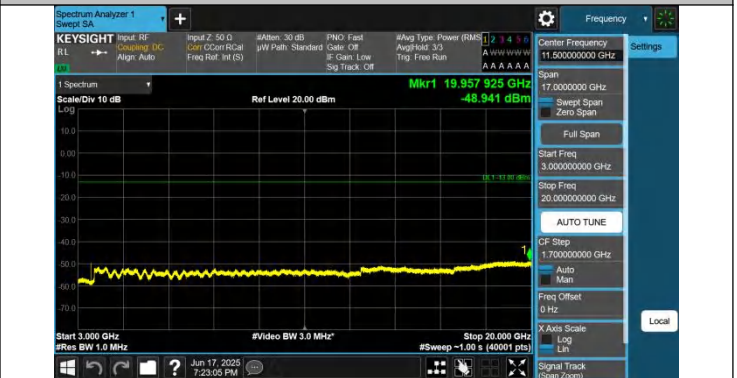
66-66-10MHz-20MHz-QPSK-QPSK-132328-132472-1RB#0-0RB #0-3000~20000MHz-PASS
