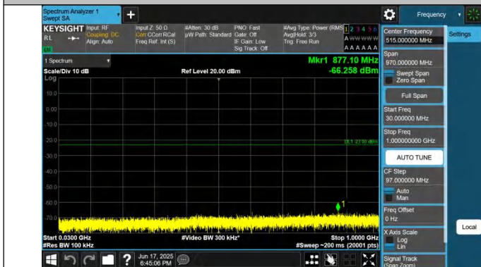
66-66-5MHz-20MHz-QPSK-QPSK-132027-132171-1RB#24-0RB #0-30~1000MHz-PASS
