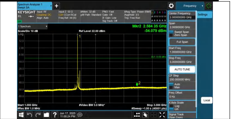
66-66-20MHz-15MHz-QPSK-QPSK-132423-132594-1RB#0-0RB #0-1000~3000MHz-PASS
