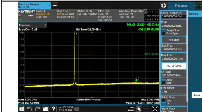
66-66-10MHz-20MHz-QPSK-QPSK-132328-132472-1RB#0-0RB #0-1000~3000MHz-PASS
