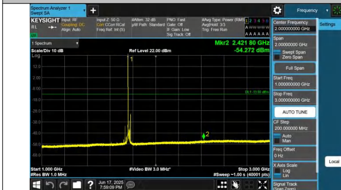
66-66-15MHz-10MHz-QPSK-QPSK-132499-132619-1RB#0-0RB #0-1000~3000MHz-PASS
