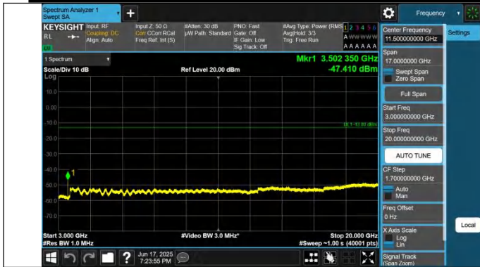
66-66-10MHz-20MHz-QPSK-QPSK-132428-132572-1RB#0-0RB #0-3000~20000MHz-PASS
