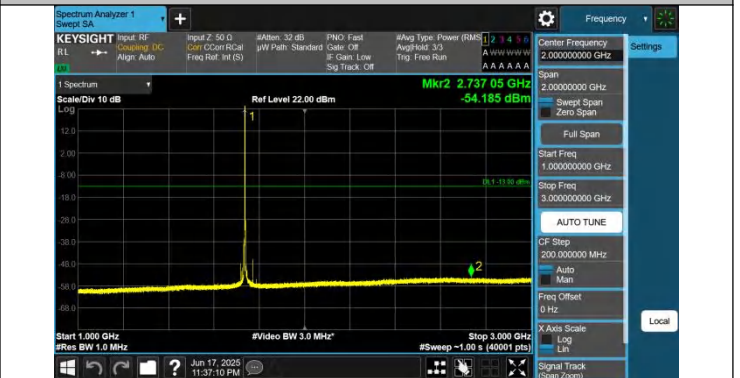
66-66-20MHz-20MHz-QPSK-QPSK-132323-132521-1RB#0-0RB #0-1000~3000MHz-PASS
