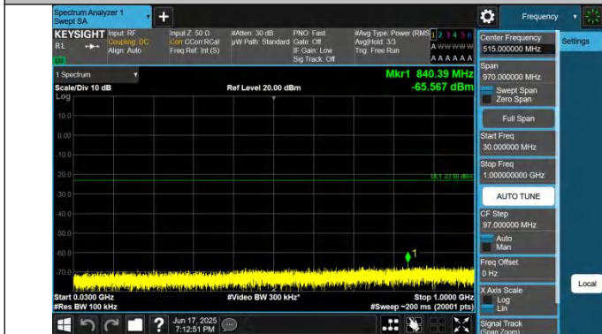
66-66-10MHz-15MHz-QPSK-QPSK-132351-132471-1RB#0-0RB #0-30~1000MHz-PASS
