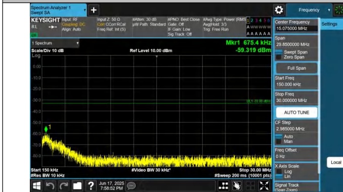
66-66-15MHz-10MHz-QPSK-QPSK-132499-132619-1RB#0-0RB #0-0.15~30MHz-PASS
