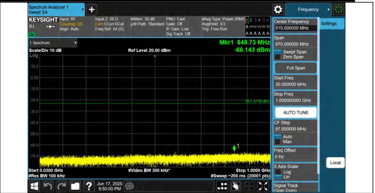
66-66-20MHz-10MHz-QPSK-QPSK-132473-132617-1RB#0-0RB #0-30~1000MHz-PASS
