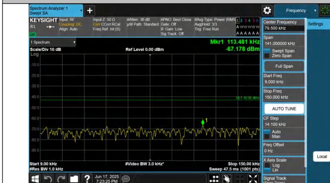
66-66-10MHz-20MHz-QPSK-QPSK-132428-132572-1RB#0-0RB #0-0.009~0.15MHz-PASS
