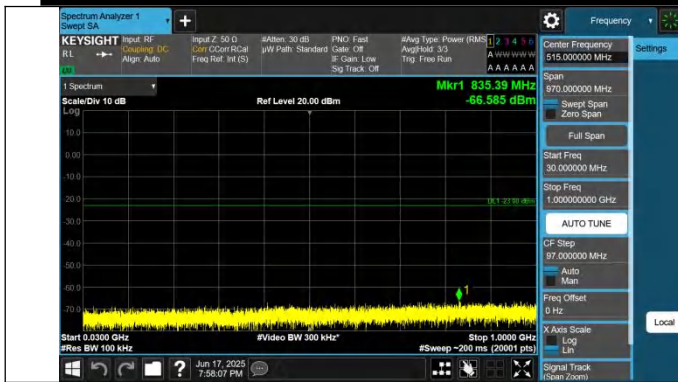
66-66-15MHz-10MHz-QPSK-QPSK-132373-132493-1RB#0-0RB #0-30~1000MHz-PASS
