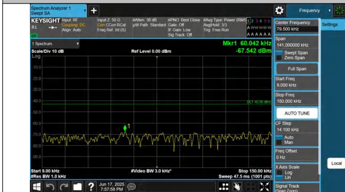
66-66-15MHz-10MHz-QPSK-QPSK-132373-132493-1RB#0-0RB #0-0.009~0.15MHz-PASS
