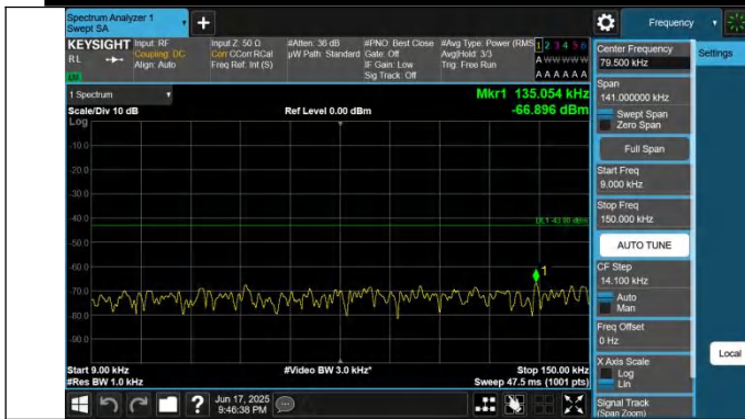
66-66-20MHz-5MHz-QPSK-QPSK-132522-132639-1RB#0-0RB# 0-0.009~0.15MHz-PASS
