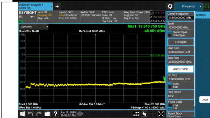
66-66-20MHz-15MHz-QPSK-QPSK-132072-132243-1RB#0-0RB #0-3000~20000MHz-PASS
