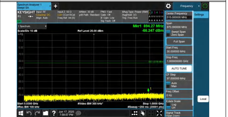
66-66-15MHz-10MHz-QPSK-QPSK-132499-132619-1RB#0-0RB #0-30~1000MHz-PASS
