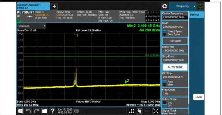
66-66-5MHz-20MHz-QPSK-QPSK-132428-132572-1RB#0-0RB# 0-1000~3000MHz-PASS
