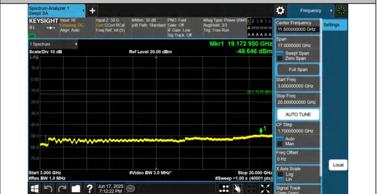
66-66-10MHz-15MHz-QPSK-QPSK-132025-132145-1RB#0-0RB #0-3000~20000MHz-PASS
