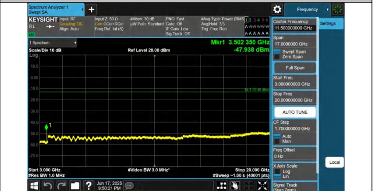
66-66-20MHz-10MHz-QPSK-QPSK-132473-132617-1RB#0-0RB #0-3000~20000MHz-PASS
