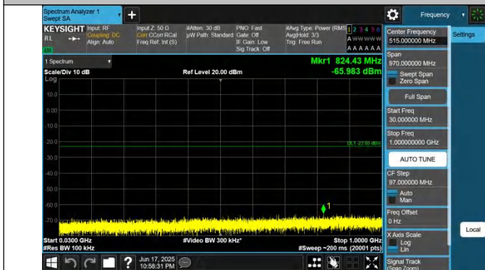
66-66-20MHz-15MHz-QPSK-QPSK-132072-132243-1RB#0-0RB #0-30~1000MHz-PASS
