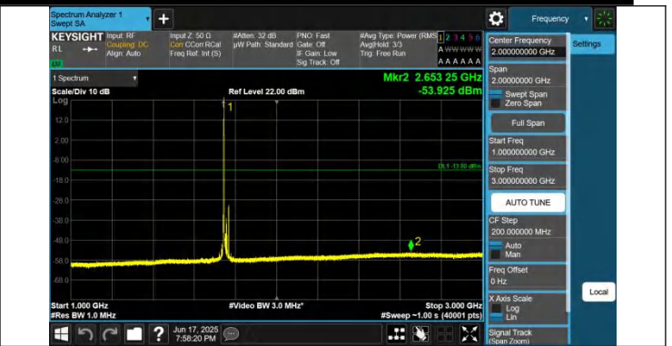
66-66-15MHz-10MHz-QPSK-QPSK-132373-132493-1RB#0-0RB #0-1000~3000MHz-PASS
