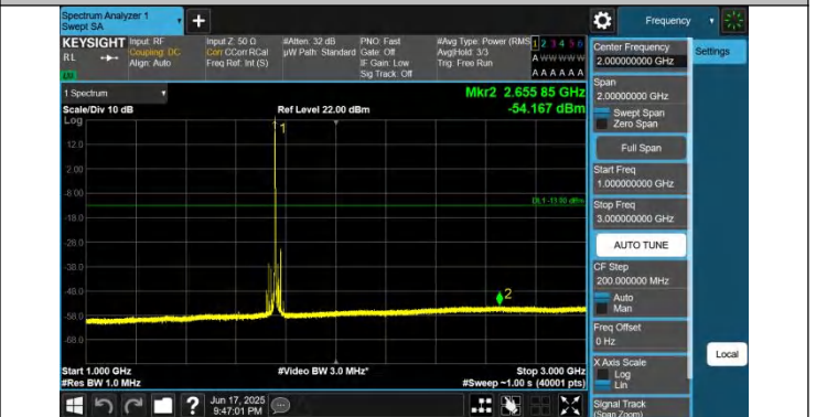
66-66-20MHz-5MHz-QPSK-QPSK-132522-132639-1RB#0-0RB# 0-1000~3000MHz-PASS
