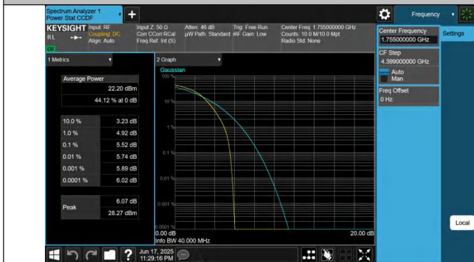
66-66-20MHz-20MHz-QPSK-QPSK-132323-132521-100RB#0-100 RB#0-PASS
