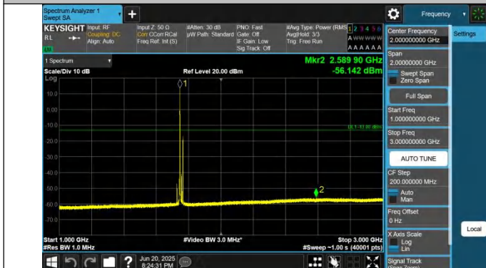
66-66-10MHz-10MHz-QPSK-QPSK-132373-132472-1RB#0-1RB #49-1000~3000MHz-PASS
