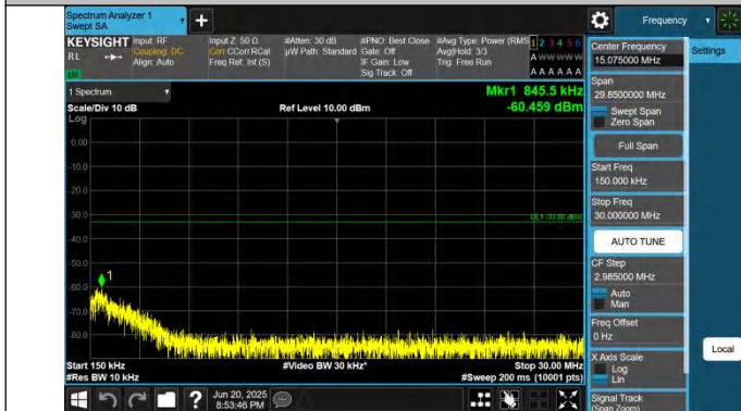
66-66-15MHz-5MHz-QPSK-QPSK-132398-132491-1RB#0-0RB# 0-0.15~30MHz-PASS
