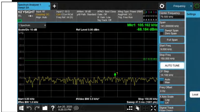
66-66-10MHz-10MHz-QPSK-QPSK-132523-132622-1RB#0-1RB #49-0.009~0.15MHz-PASS
