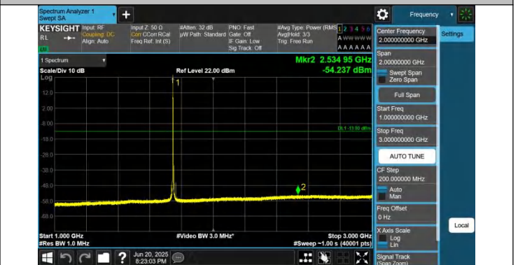
66-66-10MHz-10MHz-QPSK-QPSK-132373-132472-1RB#0-0RB #0-1000~3000MHz-PASS
