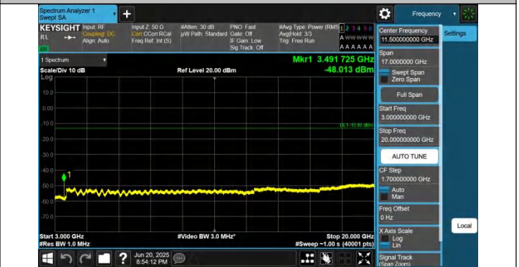
66-66-15MHz-5MHz-QPSK-QPSK-132398-132491-1RB#0-0RB# 0-3000~20000MHz-PASS
