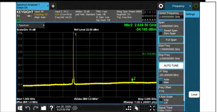
66-66-10MHz-10MHz-QPSK-QPSK-132373-132472-1RB#49-0R B#0-1000~3000MHz-PASS
