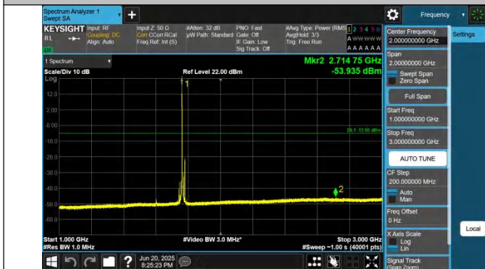
66-66-10MHz-10MHz-QPSK-QPSK-132523-132622-1RB#0-0RB #0-1000~3000MHz-PASS
