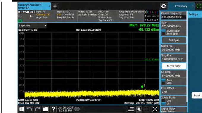
66-66-10MHz-10MHz-QPSK-QPSK-132373-132472-1RB#49-0R B#0-30~1000MHz-PASS
