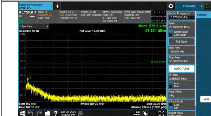
66-66-10MHz-10MHz-QPSK-QPSK-132523-132622-1RB#0-0RB #0-0.15~30MHz-PASS
