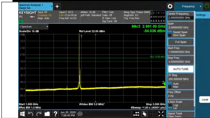
66-66-5MHz-10MHz-QPSK-QPSK-132550-132622-1RB#0-0RB# 0-1000~3000MHz-PASS
