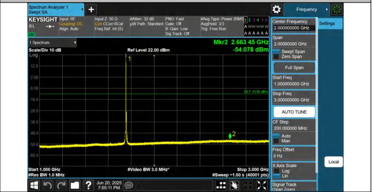
66-66-5MHz-10MHz-QPSK-QPSK-132375-132447-1RB#24-0RB #0-1000~3000MHz-PASS
