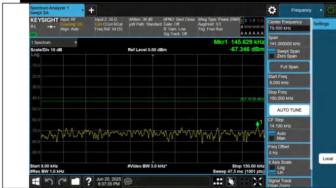
66-66-5MHz-15MHz-QPSK-QPSK-132353-132446-1RB#0-0RB# 0-0.009~0.15MHz-PASS
