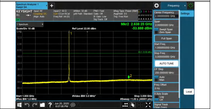
66-66-10MHz-5MHz-QPSK-QPSK-132022-132094-1RB#49-0RB #0-1000~3000MHz-PASS
