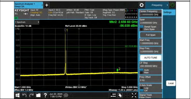
66-66-5MHz-10MHz-QPSK-QPSK-132550-132622-1RB#0-1RB# 49-1000~3000MHz-PASS
