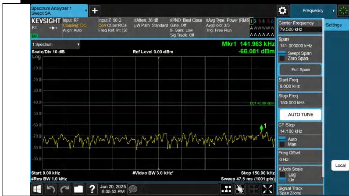
66-66-10MHz-5MHz-QPSK-QPSK-132022-132094-1RB#0-0RB# 0-0.009~0.15MHz-PASS
