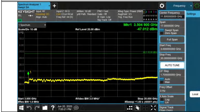
66-66-5MHz-10MHz-QPSK-QPSK-132375-132447-1RB#24-0RB #0-3000~20000MHz-PASS
