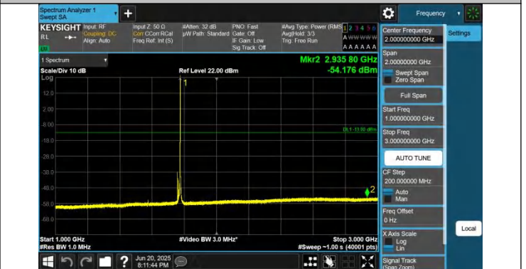
66-66-10MHz-5MHz-QPSK-QPSK-132572-132644-1RB#49-0RB #0-1000~3000MHz-PASS
