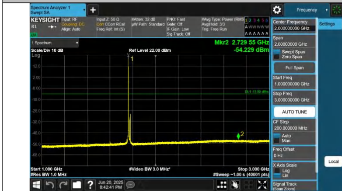
66-66-5MHz-15MHz-QPSK-QPSK-132504-132597-1RB#0-1RB# 74-1000~3000MHz-PASS
