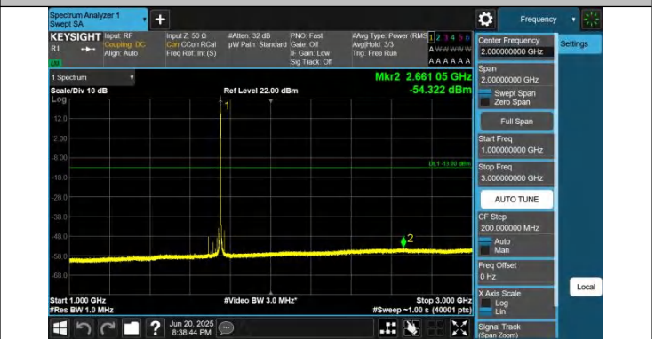
66-66-5MHz-15MHz-QPSK-QPSK-132353-132446-1RB#24-0RB #0-1000~3000MHz-PASS
