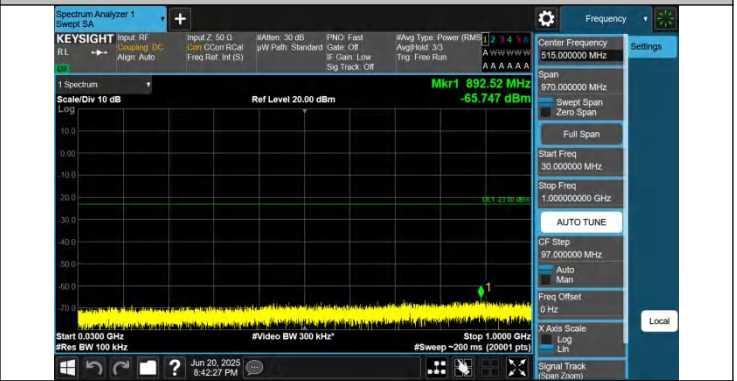
66-66-5MHz-15MHz-QPSK-QPSK-132504-132597-1RB#0-1RB# 74-30~1000MHz-PASS
