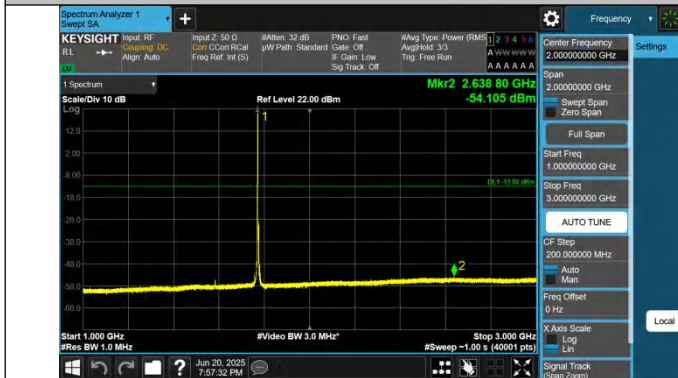
66-66-5MHz-10MHz-QPSK-QPSK-132550-132622-1RB#24-0RB #0-1000~3000MHz-PASS
