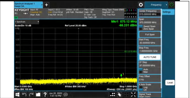
66-66-5MHz-10MHz-QPSK-QPSK-132550-132622-1RB#24-0RB #0-30~1000MHz-PASS
