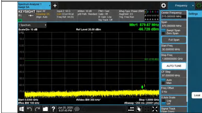
66-66-5MHz-15MHz-QPSK-QPSK-132353-132446-1RB#0-0RB# 0-30~1000MHz-PASS
