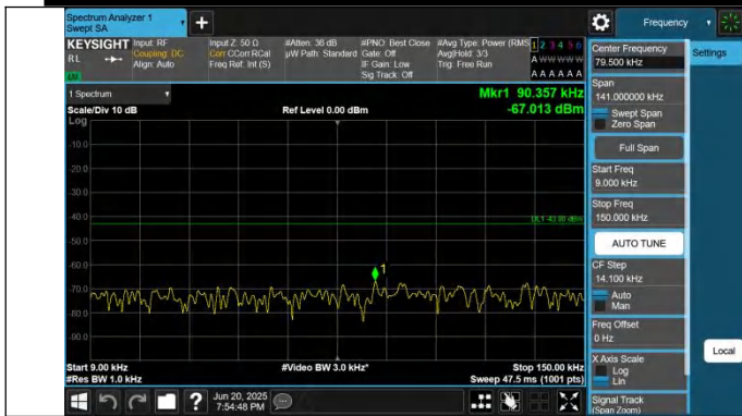
66-66-5MHz-10MHz-QPSK-QPSK-132375-132447-1RB#24-0RB #0-0.009~0.15MHz-PASS
