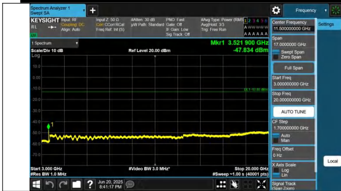
66-66-5MHz-15MHz-QPSK-QPSK-132504-132597-1RB#0-0RB# 0-3000~20000MHz-PASS
