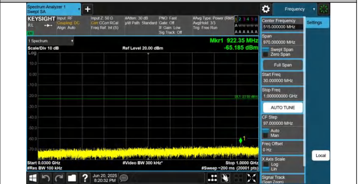
66-66-10MHz-10MHz-QPSK-QPSK-132022-132121-1RB#0-0RB #0-30~1000MHz-PASS
