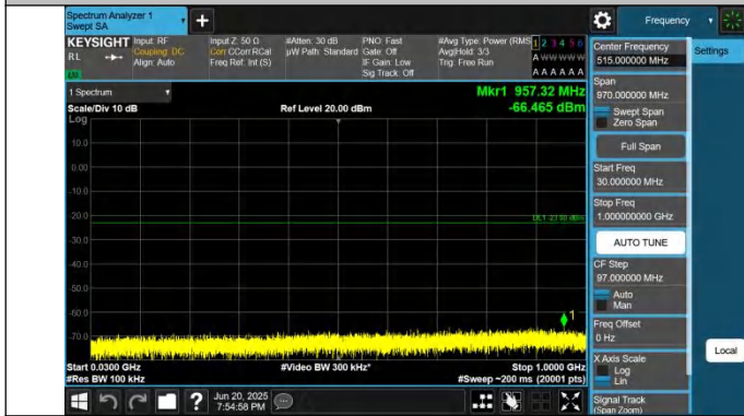
66-66-5MHz-10MHz-QPSK-QPSK-132375-132447-1RB#24-0RB #0-30~1000MHz-PASS
