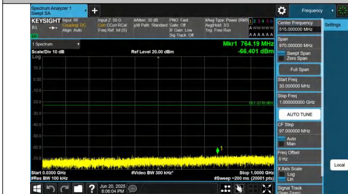
66-66-10MHz-5MHz-QPSK-QPSK-132022-132094-1RB#0-0RB# 0-30~1000MHz-PASS
