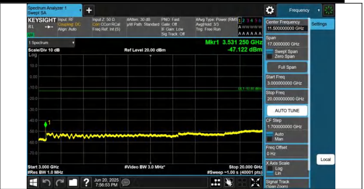
66-66-5MHz-10MHz-QPSK-QPSK-132550-132622-1RB#0-0RB# 0-3000~20000MHz-PASS
