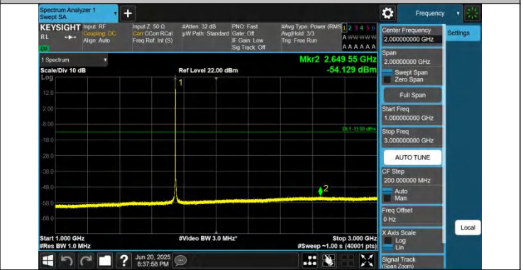
66-66-5MHz-15MHz-QPSK-QPSK-132353-132446-1RB#0-0RB# 0-1000~3000MHz-PASS
