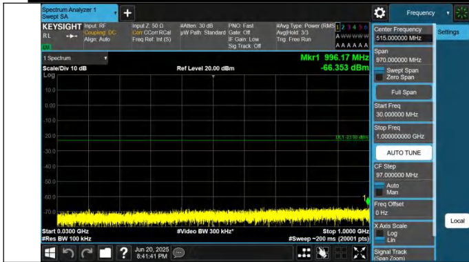
66-66-5MHz-15MHz-QPSK-QPSK-132504-132597-1RB#24-0RB #0-30~1000MHz-PASS
