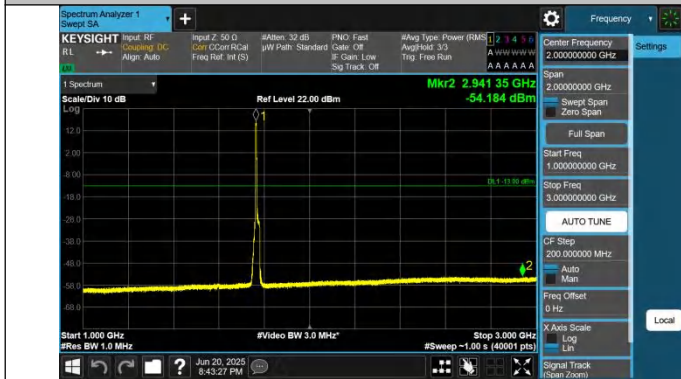
66-66-5MHz-15MHz-QPSK-QPSK-132504-132597-25RB#0-75R B#0-1000~3000MHz-PASS
