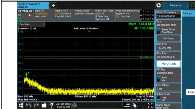
66-66-10MHz-10MHz-QPSK-QPSK-132022-132121-1RB#0-0RB #0-0.15~30MHz-PASS
