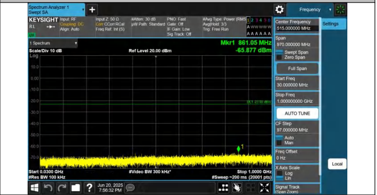
66-66-5MHz-10MHz-QPSK-QPSK-132550-132622-1RB#0-0RB# 0-30~1000MHz-PASS
