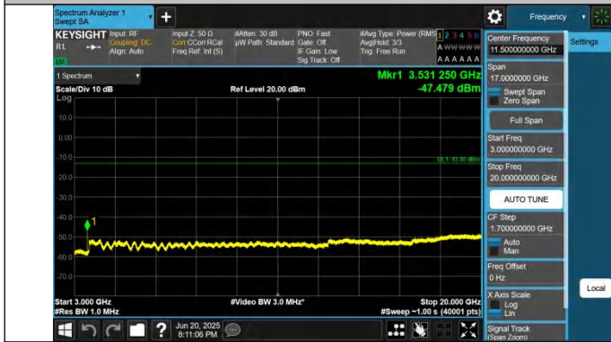
66-66-10MHz-5MHz-QPSK-QPSK-132572-132644-1RB#0-0RB# 0-3000~20000MHz-PASS
