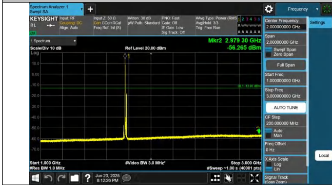
66-66-10MHz-5MHz-QPSK-QPSK-132572-132644-1RB#0-1RB# 24-1000~3000MHz-PASS
