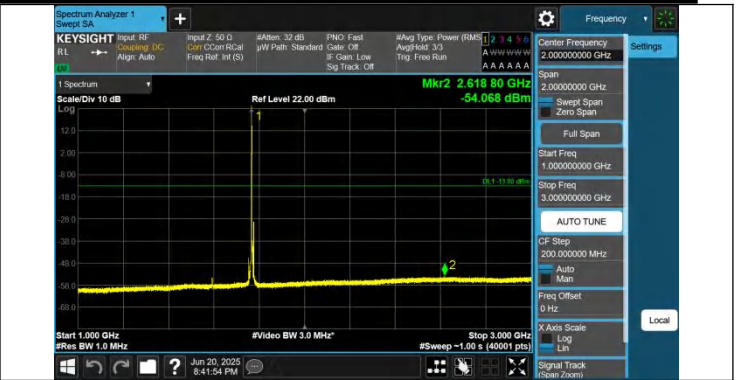
66-66-5MHz-15MHz-QPSK-QPSK-132504-132597-1RB#24-0RB #0-1000~3000MHz-PASS
