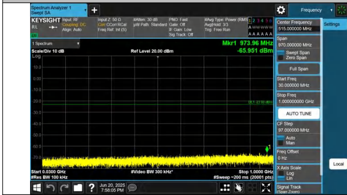
66-66-5MHz-10MHz-QPSK-QPSK-132550-132622-1RB#0-1RB# 49-30~1000MHz-PASS
