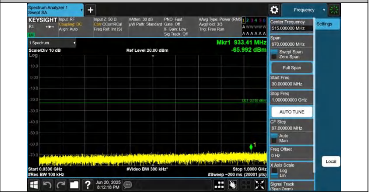
66-66-10MHz-5MHz-QPSK-QPSK-132572-132644-1RB#0-1RB# 24-30~1000MHz-PASS
