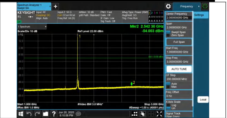
66-66-10MHz-5MHz-QPSK-QPSK-132572-132644-1RB#0-0RB# 0-1000~3000MHz-PASS
