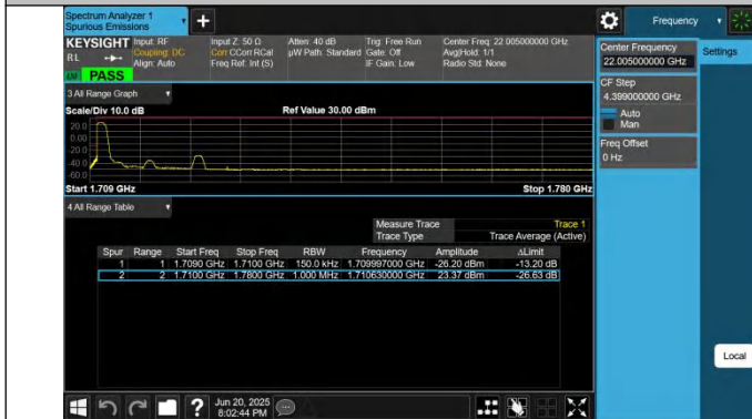
66-66-10MHz-5MHz-QPSK@QPSK-QPSK@QPSK-132022-1320 94-1RB#0@50RB#0-0RB#0@25RB#0-PASS
