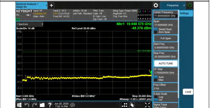
66-66-5MHz-10MHz-QPSK-QPSK-132000-132072-1RB#0-0RB# 0-3000~20000MHz-PASS
