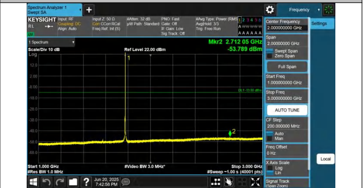
66-66-5MHz-5MHz-QPSK-QPSK-132599-132647-1RB#24-0RB# 0-1000~3000MHz-PASS
