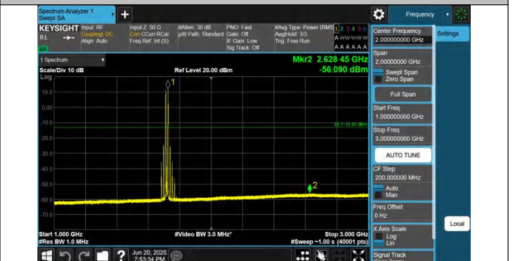
66-66-5MHz-10MHz-QPSK-QPSK-132000-132072-1RB#0-1RB# 49-1000~3000MHz-PASS
