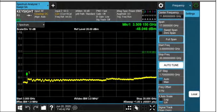
66-66-5MHz-5MHz-QPSK-QPSK-132398-132446-1RB#24-0RB# 0-3000~20000MHz-PASS
