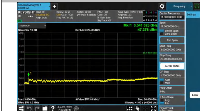
66-66-5MHz-5MHz-QPSK-QPSK-132599-132647-1RB#0-0RB#0- 3000~20000MHz-PASS
