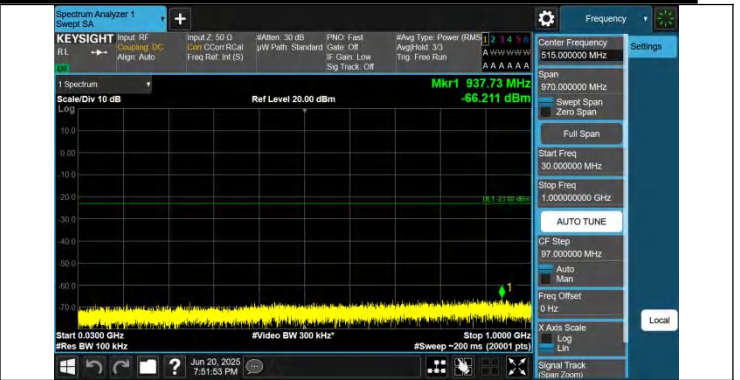
66-66-5MHz-10MHz-QPSK-QPSK-132000-132072-1RB#0-0RB# 0-30~1000MHz-PASS
