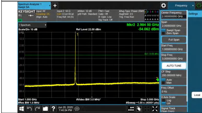
66-66-5MHz-5MHz-QPSK-QPSK-132398-132446-1RB#24-0RB# 0-1000~3000MHz-PASS
