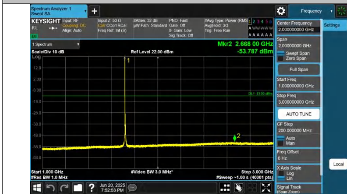
66-66-5MHz-10MHz-QPSK-QPSK-132000-132072-1RB#24-0RB #0-1000~3000MHz-PASS
