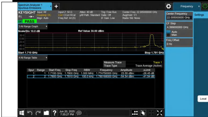
66-66-5MHz-5MHz-QPSK@QPSK-QPSK@QPSK-132599-13264 7-1RB#24@25RB#0-0RB#0@25RB#0-PASS
