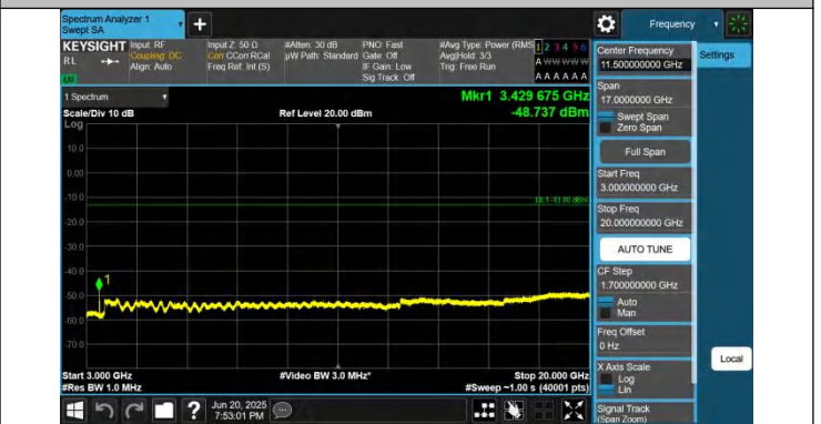
66-66-5MHz-10MHz-QPSK-QPSK-132000-132072-1RB#24-0RB #0-3000~20000MHz-PASS
