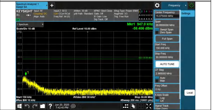
66-66-5MHz-5MHz-QPSK-QPSK-132599-132647-1RB#24-0RB# 0-0.15~30MHz-PASS
