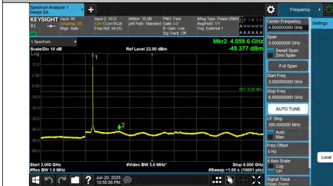
43-43-20MHz-20MHz-QPSK-QPSK-44690-44888-1RB#0-0RB#0- 3000~6000MHz-PASS
