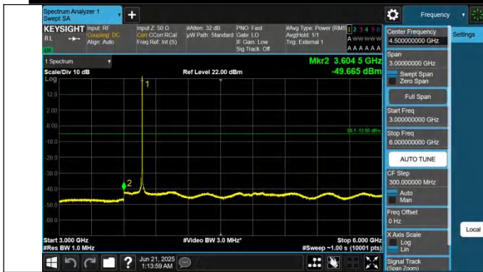
43-43-20MHz-10MHz-QPSK-QPSK-45391-45535-1RB#0-0RB#0-3000~6000MHz-PASS
