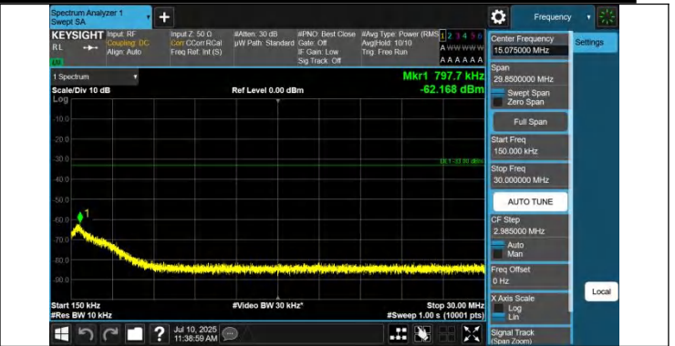
43-43-20MHz-20MHz-QPSK-QPSK-44690-44888-1RB#0-0RB#0- 0.15~30MHz-PASS
