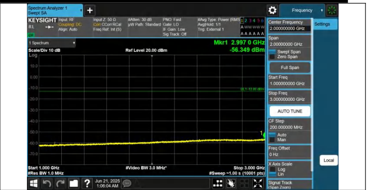
43-43-20MHz-10MHz-QPSK-QPSK-44690-44834-1RB#0-0RB#0-1000~3000MHz-PASS
