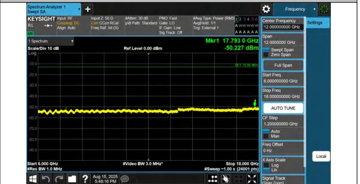
43-43-20MHz-20MHz-QPSK-QPSK-45292-45490-1RB#0-0RB#0- 6000~18000MHz-PASS
