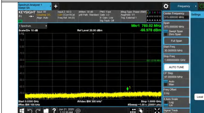
43-43-20MHz-10MHz-QPSK-QPSK-45391-45535-1RB#0-0RB#0-30~1000MHz-PASS
