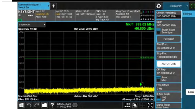
43-43-20MHz-20MHz-QPSK-QPSK-45292-45490-1RB#0-0RB#0- 30~1000MHz-PASS
