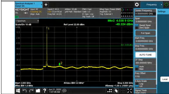
43-43-20MHz-10MHz-QPSK-QPSK-44690-44834-1RB#0-0RB#0-3000~6000MHz-PASS
