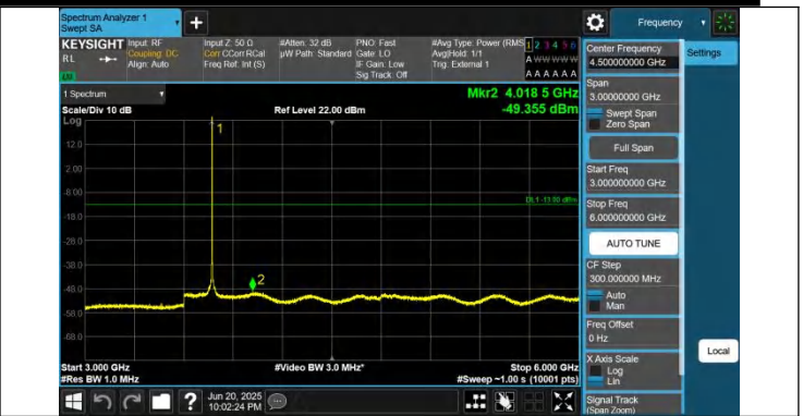
43-43-10MHz-20MHz-QPSK-QPSK-45346-45490-1RB#0-0RB#0-3000~6000MHz-PASS
