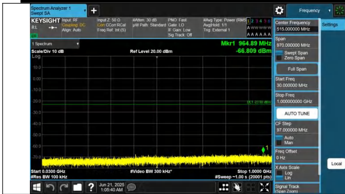
43-43-20MHz-10MHz-QPSK-QPSK-44690-44834-1RB#0-0RB#0-30~1000MHz-PASS
