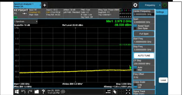
43-43-20MHz-20MHz-QPSK-QPSK-45292-45490-1RB#0-0RB#0- 1000~3000MHz-PASS
