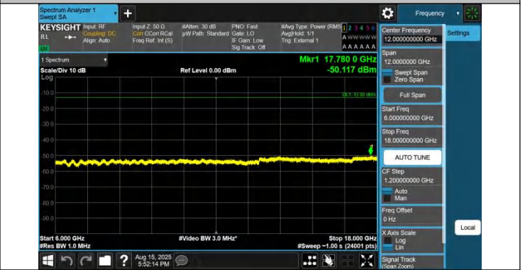
43-43-20MHz-10MHz-QPSK-QPSK-44690-44834-1RB#0-0RB#0-6000~18000MHz-PASS
