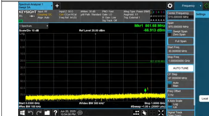
43-43-20MHz-20MHz-QPSK-QPSK-44690-44888-1RB#0-0RB#0- 30~1000MHz-PASS
