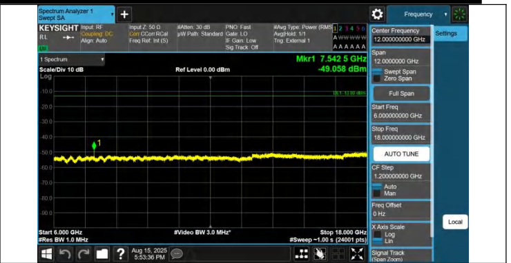
43-43-20MHz-10MHz-QPSK-QPSK-45391-45535-1RB#0-0RB#0-6000~18000MHz-PASS
