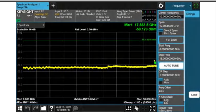
43-43-20MHz-20MHz-QPSK-QPSK-44690-44888-1RB#0-0RB#0- 6000~18000MHz-PASS
