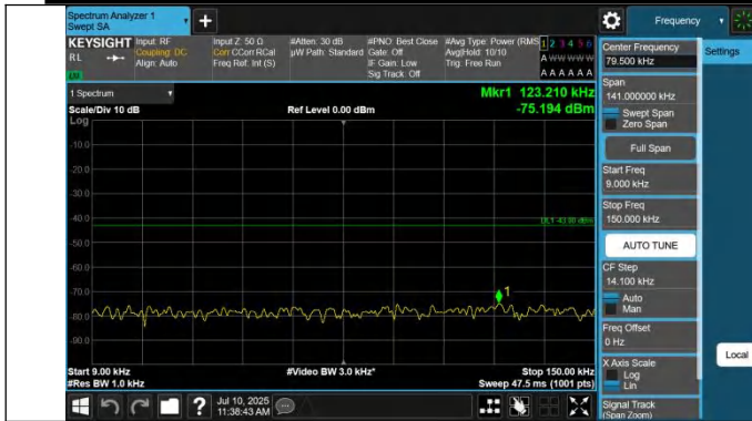
43-43-20MHz-20MHz-QPSK-QPSK-44690-44888-1RB#0-0RB#0- 0.009~0.15MHz-PASS
