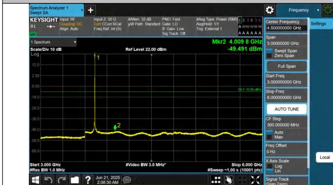
43-43-20MHz-15MHz-QPSK-QPSK-45016-45187-1RB#0-0RB#0-3000~6000MHz-PASS
