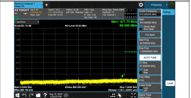
43-43-5MHz-20MHz-QPSK-QPSK-44998-45115-1RB#0-0RB#0-3 0~1000MHz-PASS
