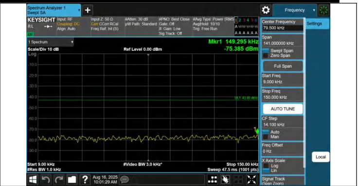
43-43-5MHz-20MHz-QPSK-QPSK-44998-45115-1RB#0-0RB#0-0. 009~0.15MHz-PASS
