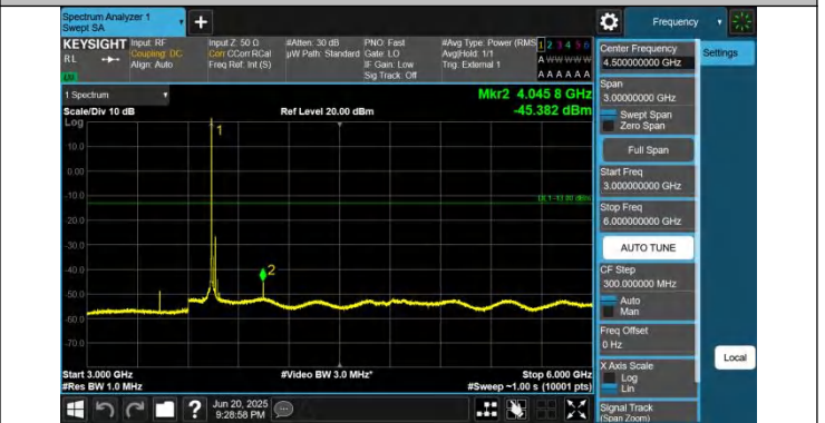
43-43-5MHz-20MHz-QPSK-QPSK-44998-45115-1RB#0-0RB#0-3 000~6000MHz-PASS
