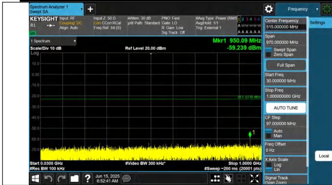
42-42-20MHz-20MHz-QPSK-QPSK-42792-42990-1RB#0-0RB#0- 30~1000MHz-PASS
