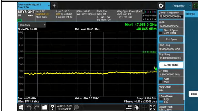
42-42-10MHz-20MHz-QPSK-QPSK-42145-42289-1RB#0-0RB#0-6000~18000MHz-PASS
