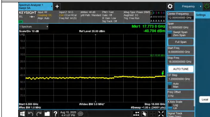
42-42-5MHz-20MHz-QPSK-QPSK-42498-42615-1RB#0-0RB#0-6 000~18000MHz-PASS
