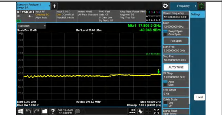
42-42-5MHz-20MHz-QPSK-QPSK-42873-42990-1RB#0-0RB#0-6 000~18000MHz-PASS
