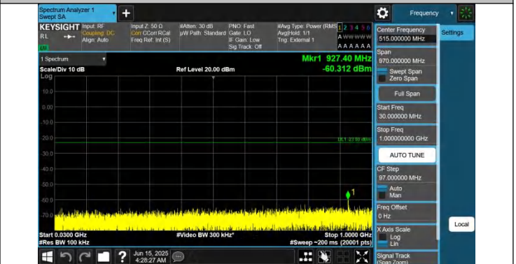
42-42-5MHz-20MHz-QPSK-QPSK-42498-42615-1RB#0-0RB#0-3 0~1000MHz-PASS
