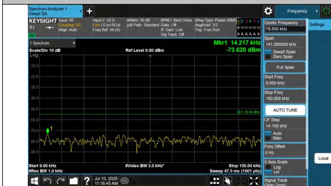
41-41-10MHz-20MHz-QPSK-QPSK-39705-39849-1RB#0-0RB#0 -0.009~0.15MHz-PASS
