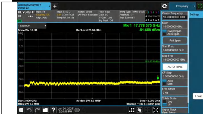
41-41-10MHz-20MHz-QPSK-QPSK-40526-40670-1RB#0-0RB#0 -3000~18000MHz-PASS
