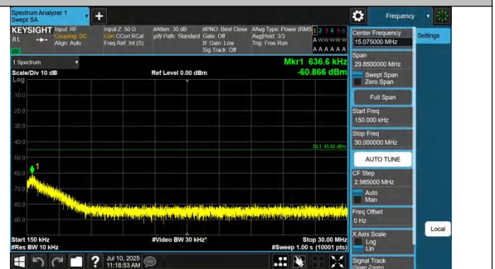
41-41-10MHz-20MHz-QPSK-QPSK-39705-39849-1RB#0-0RB#0- 0.15~30MHz-PASS
