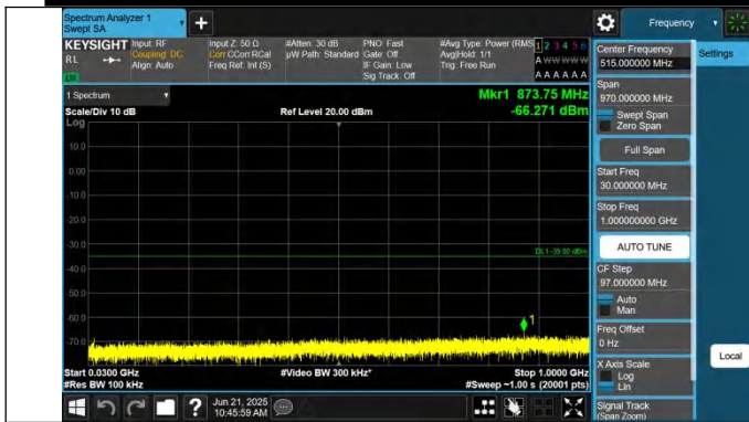
0~1000MHz-PASS
