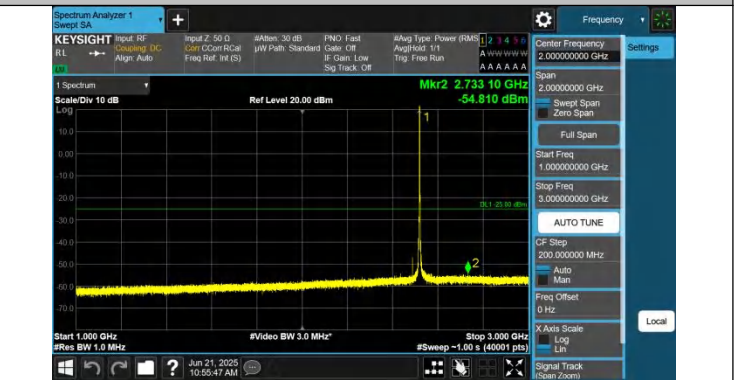
7-7-20MHz-15MHz-QPSK-QPSK-21026-21197-1RB#0-0RB#0-10 00~3000MHz-PASS
