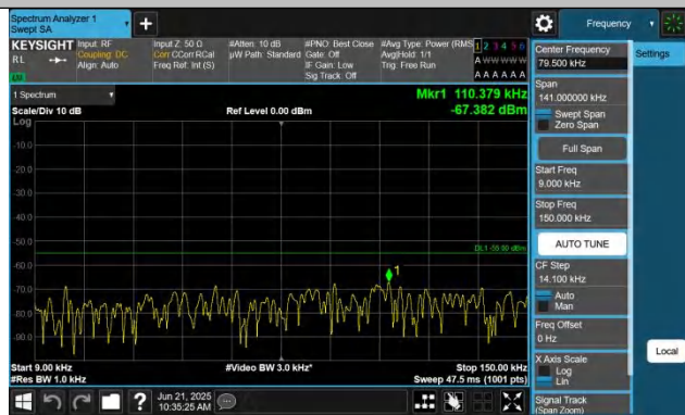
7-7-15MHz-20MHz-QPSK-QPSK-21179-21350-1RB#0-0RB#0-0. 009~0.15MHz-PASS
