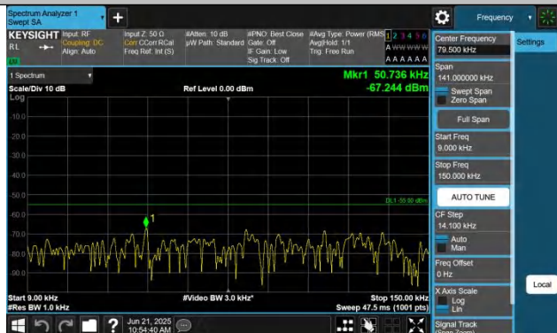
009~0.15MHz-PASS
