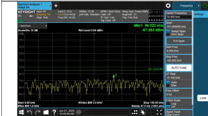
7-7-20MHz-10MHz-QPSK-QPSK-21251-21395-1RB#0-0RB#0-0. 009~0.15MHz-PASS
