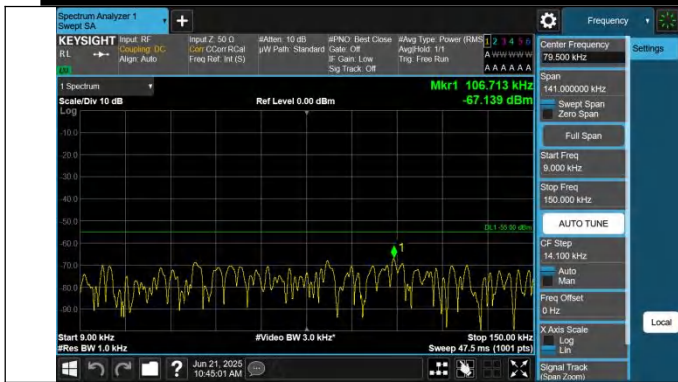
7-7-20MHz-10MHz-QPSK-QPSK-21051-21195-1RB#0-0RB#0-0. 009~0.15MHz-PASS
