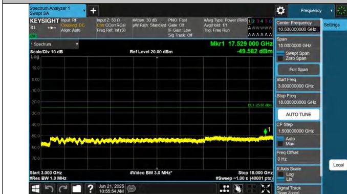
7-7-20MHz-15MHz-QPSK-QPSK-21026-21197-1RB#0-0RB#0-30 00~18000MHz-PASS
