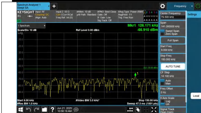
7-7-20MHz-15MHz-QPSK-QPSK-21201-21372-1RB#0-0RB#0-0. 009~0.15MHz-PASS
