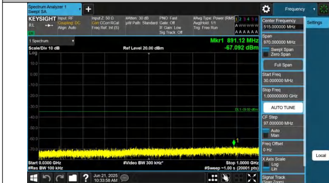
7-7-15MHz-20MHz-QPSK-QPSK-20828-20999-1RB#0-0RB#0-3 0~1000MHz-PASS
