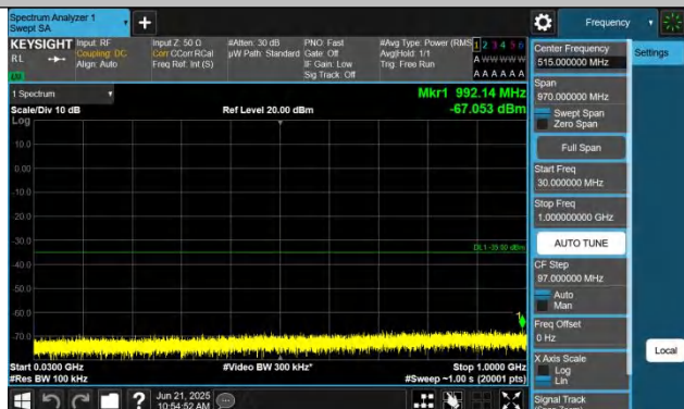
0~1000MHz-PASS
