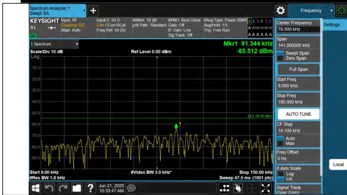
7-7-15MHz-20MHz-QPSK-QPSK-20828-20999-1RB#0-0RB#0-0. 009~0.15MHz-PASS
