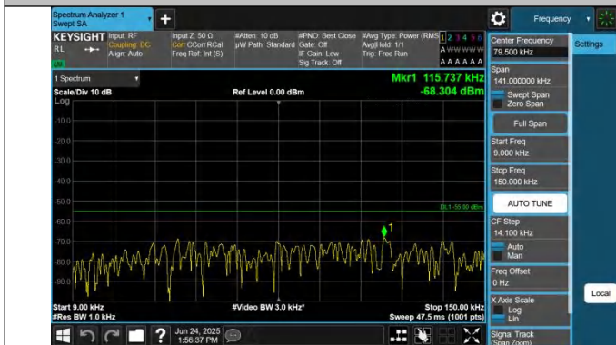
7-7-20MHz-20MHz-QPSK-QPSK-21152-21350-1RB#0-0RB#0-0. 009~0.15MHz-PASS
