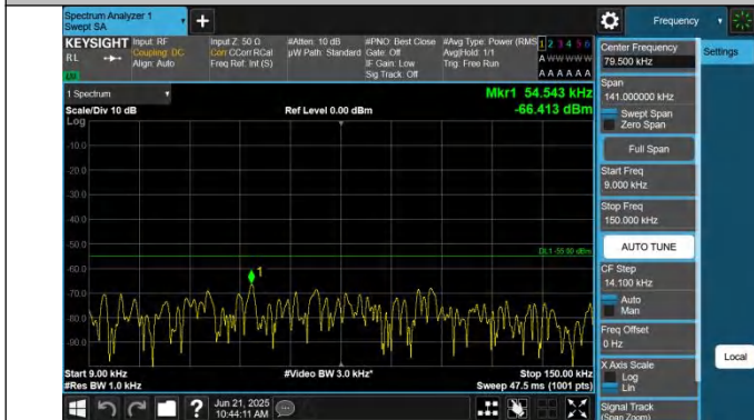
7-7-20MHz-10MHz-QPSK-QPSK-20850-20994-1RB#0-0RB#0-0. 009~0.15MHz-PASS
