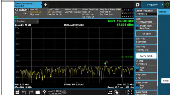
7-7-20MHz-15MHz-QPSK-QPSK-21026-21197-1RB#0-0RB#0-0. 009~0.15MHz-PASS
