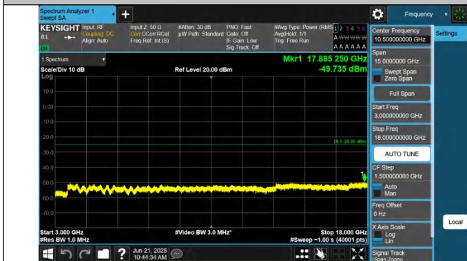
7-7-20MHz-10MHz-QPSK-QPSK-20850-20994-1RB#0-0RB#0-3 000~18000MHz-PASS
