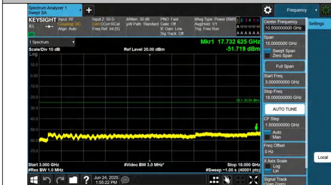
7-7-20MHz-20MHz-QPSK-QPSK-20850-21048-1RB#0-0RB#0-3 000~18000MHz-PASS
