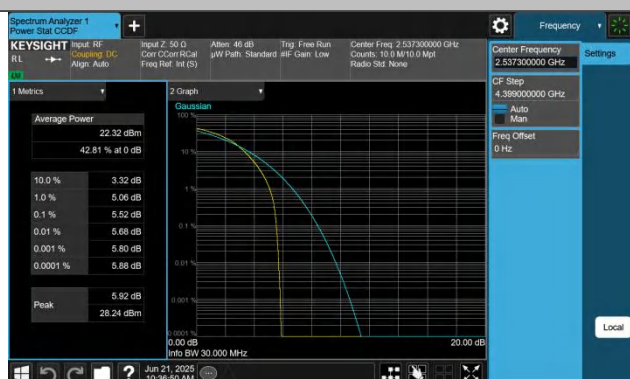
7-7-20MHz-10MHz-QPSK-QPSK-21051-21195-100RB#0-50RB#0-
