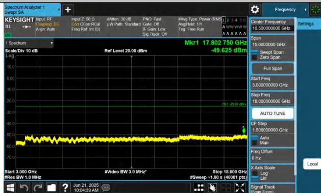
7-7-10MHz-20MHz-QPSK-QPSK-21206-21350-1RB#0-0RB#0-3 000~18000MHz-PASS
