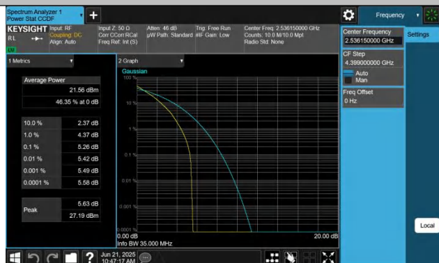
7-7-20MHz-15MHz-QPSK-QPSK-21026-21197-100RB#0-75RB#0-
