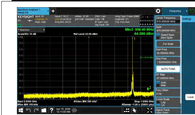
5-5-3MHz-5MHz-QPSK-QPSK-20586-20625-1RB#0-ORB#0-30~1 000MHz-PASS
