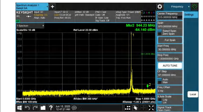
5-5-5MHz-3MHz-QPSK-QPSK-20425-20464-1RB#0-ORB#0-30~1 000MHz-PASS
