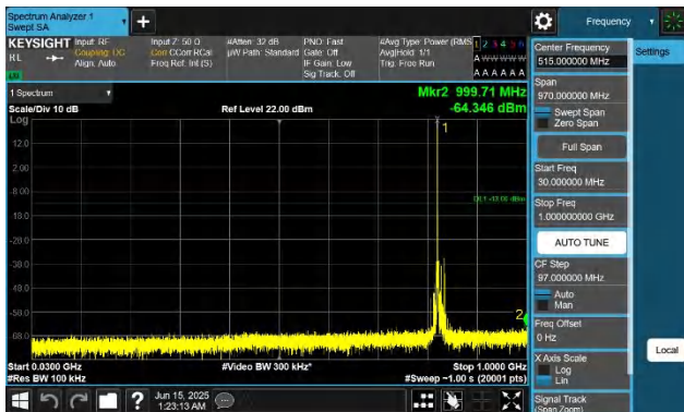
5-5-5MHz-10MHz-QPSK-QPSK-20428-20500-1RB#0-ORB#0-30~ 1000MHz-PASS
