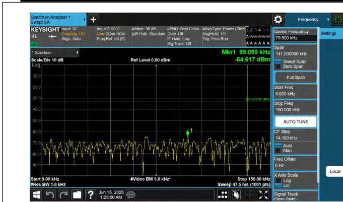
5-5-5MHz-10MHz-QPSK-QPSK-20428-20500-1RB#0-ORB#0-0.0 09~0.15MHz-PASS
