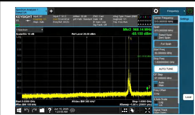
5-5-5MHz-10MHz-QPSK-QPSK-20478-20550-1RB#0-ORB#0-30~ 1000MHz-PASS
