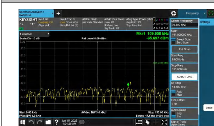
5-5-5MHz-10MHz-QPSK-QPSK-20528-20600-1RB#0-ORB#0-0.0 09~0.15MHz-PASS
