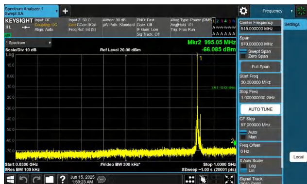
5-5-10MHz-5MHz-QPSK-QPSK-20500-20572-1RB#0-0RB#0-30~ 1000MHz-PASS
