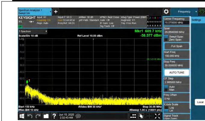
5-5-10MHz-10MHz-QPSK-QPSK-20476-20575-1RB#0-ORB#0-0. 15~30MHz-PASS
