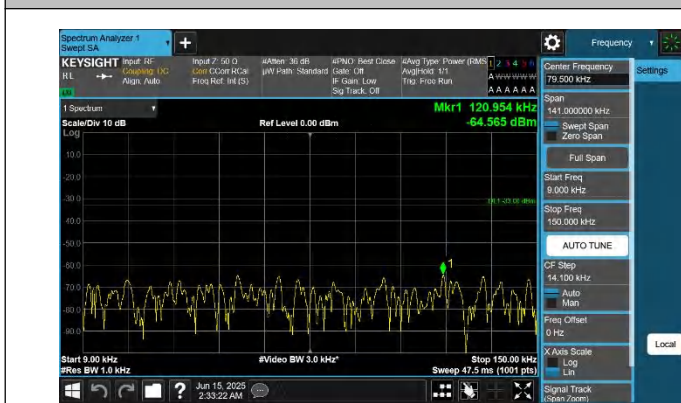
5-5-10MHz-10MHz-QPSK-QPSK-20501-20600-1RB#0-ORB#0-0. 009~0.15MHz-PASS
